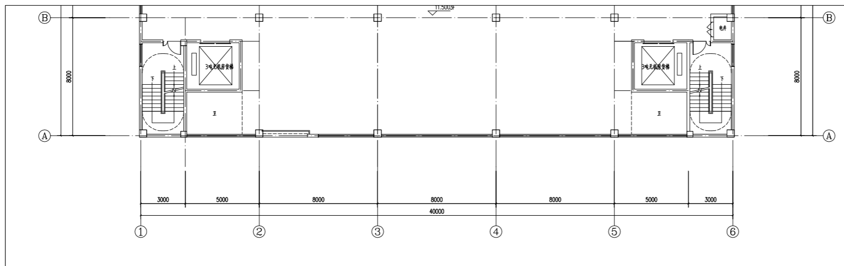
B53#三至五层平面图 1:100
