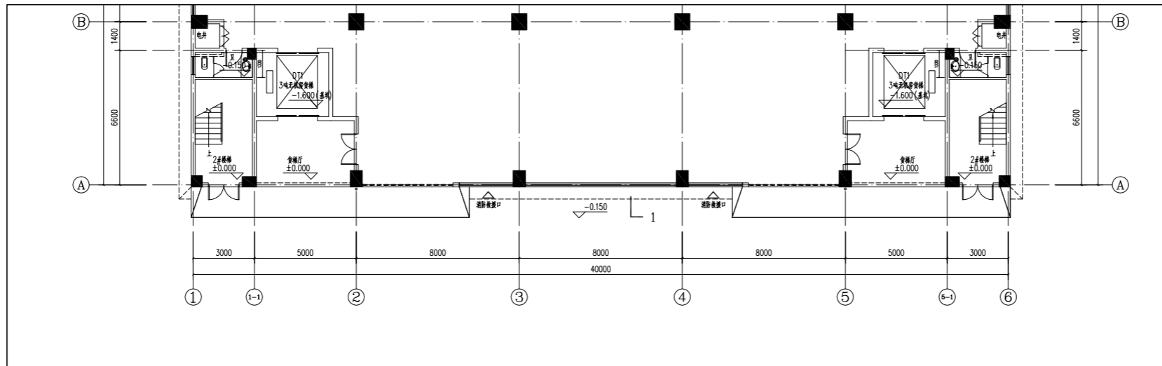
B53#一层平面图 1:100
