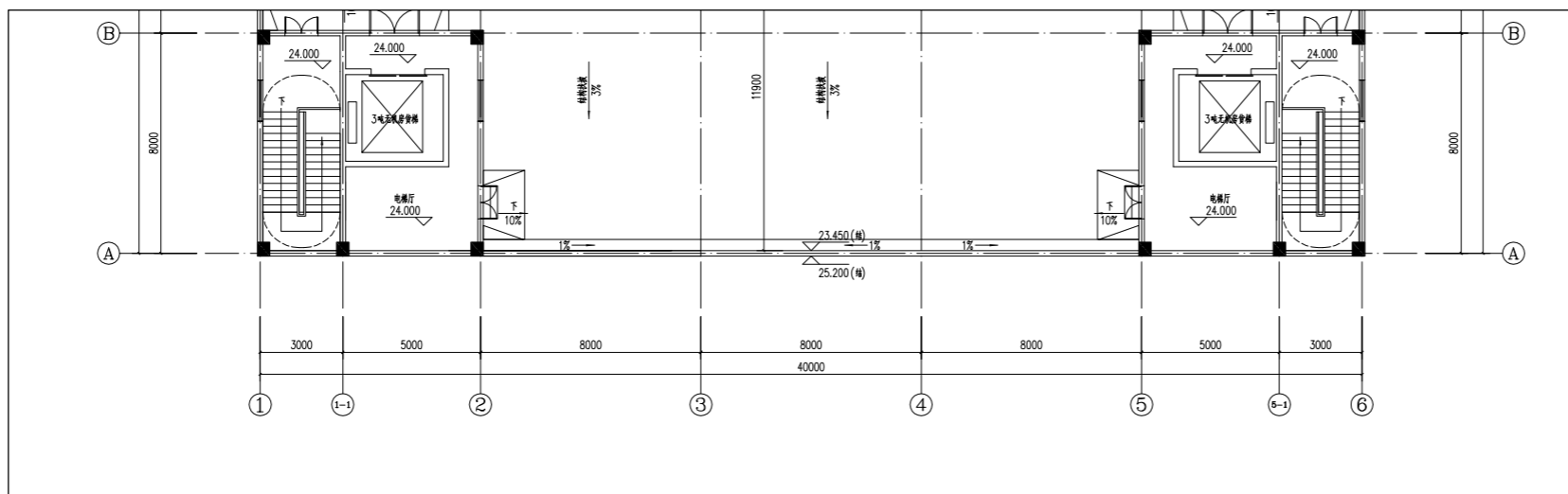
B55#屋顶层平面图 1:100
