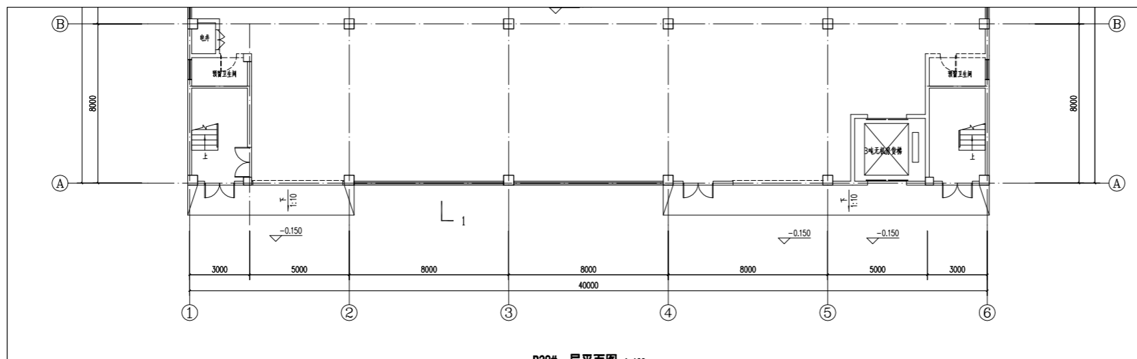
B38#一层平面图 1:100
