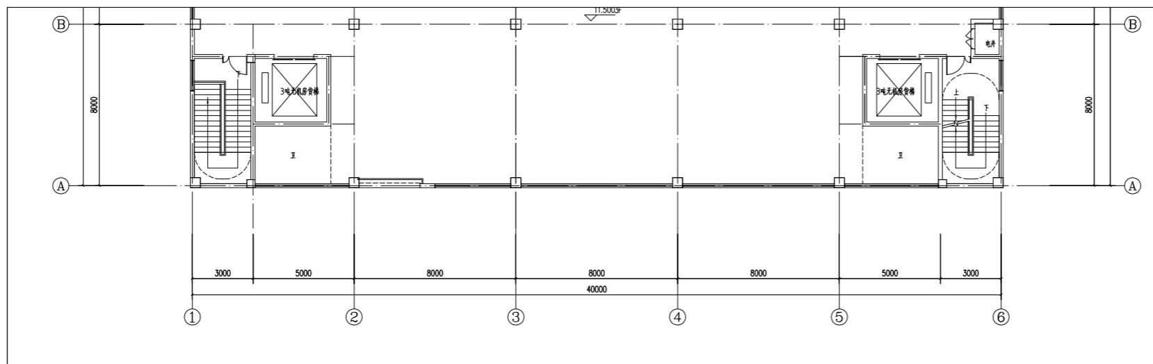
B55#三至五层平面图 1:100
