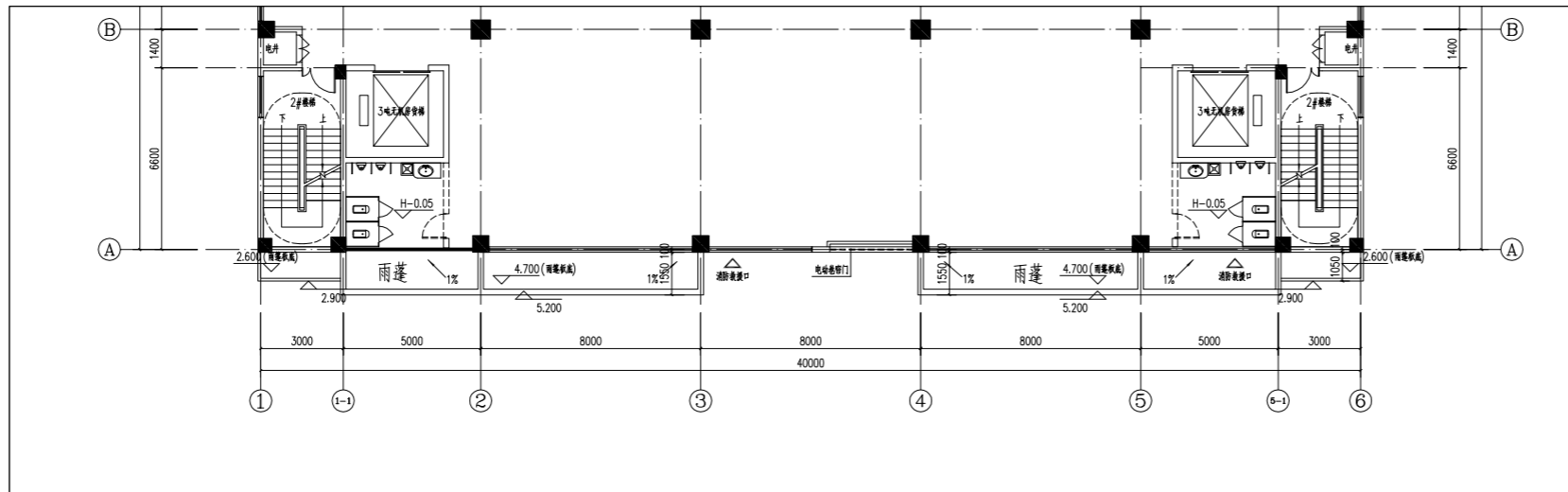
B53#二层平面图 1:100
