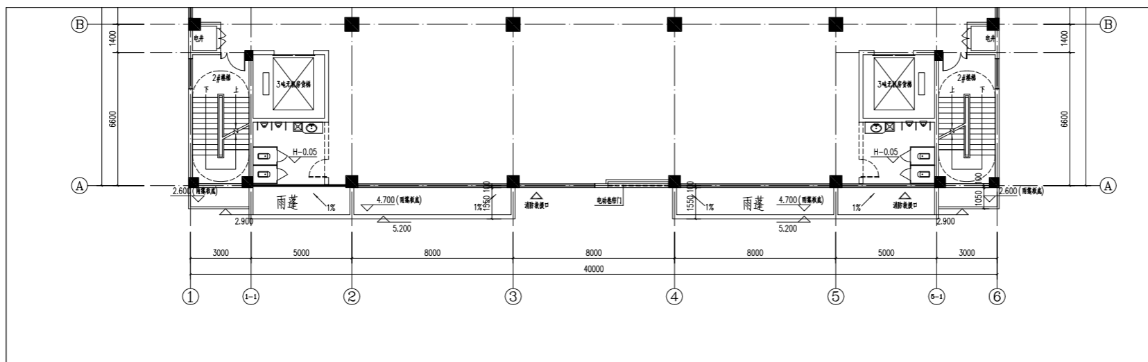
B55#二层平面图 1:100
