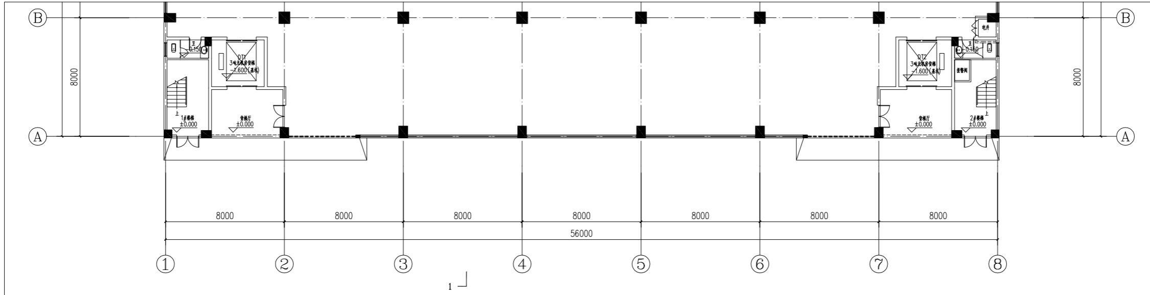
B59#一层平面图 1:100
