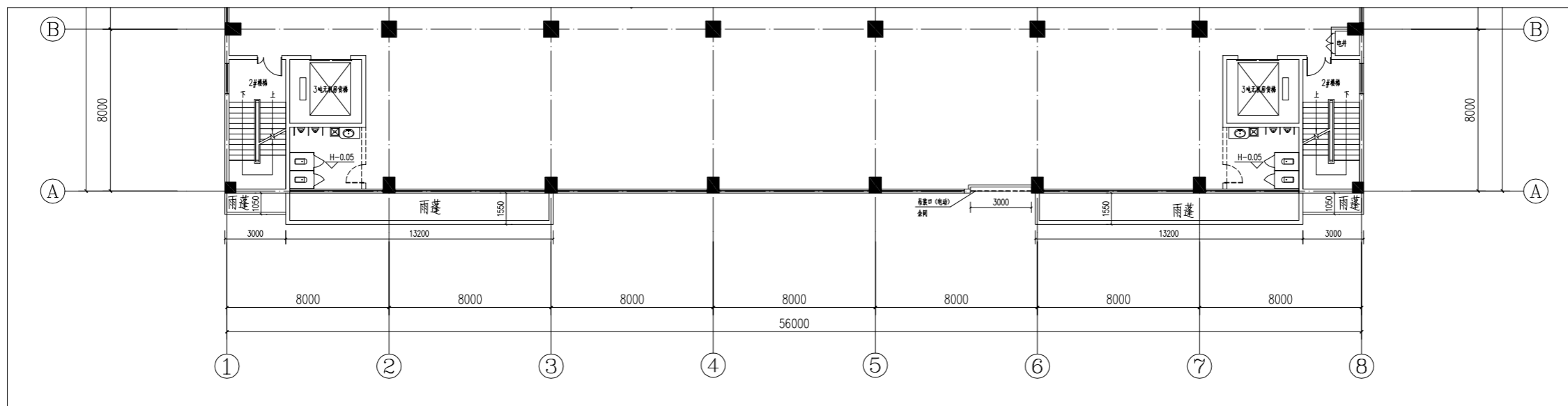
B60#二层平面图 1:100
