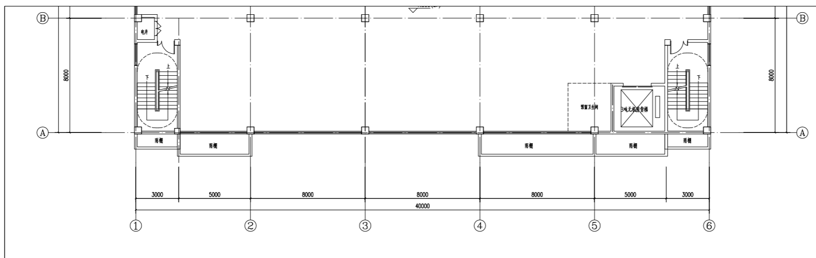
B38#二层平面图 1:100
