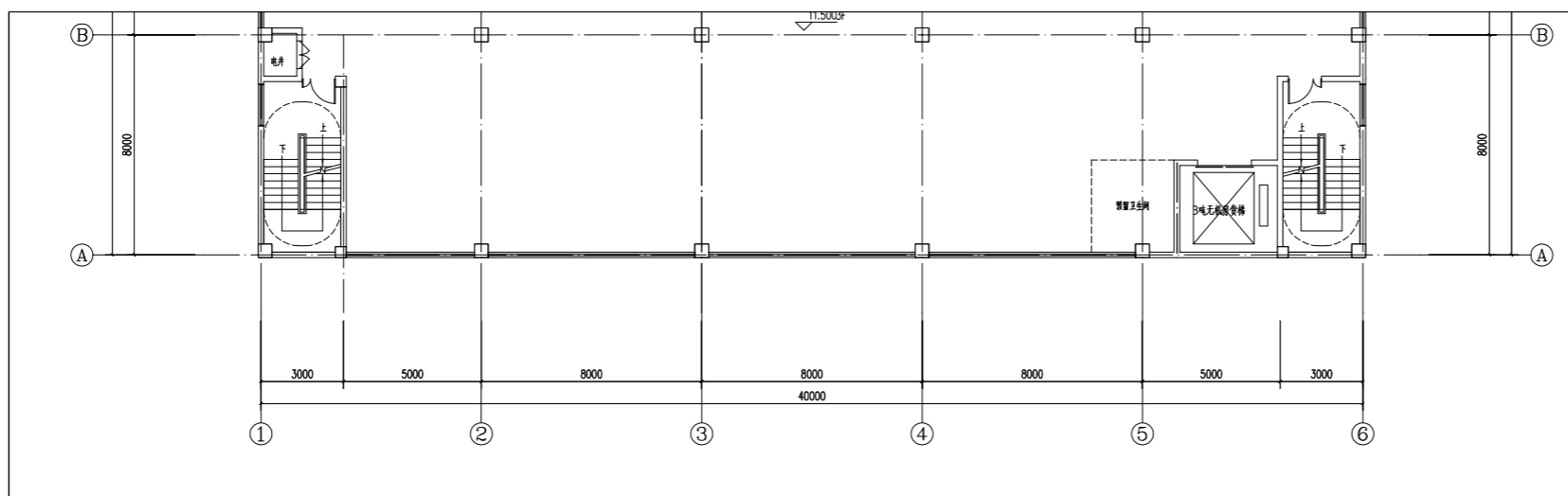
B38#三至五层平面图 1:100
