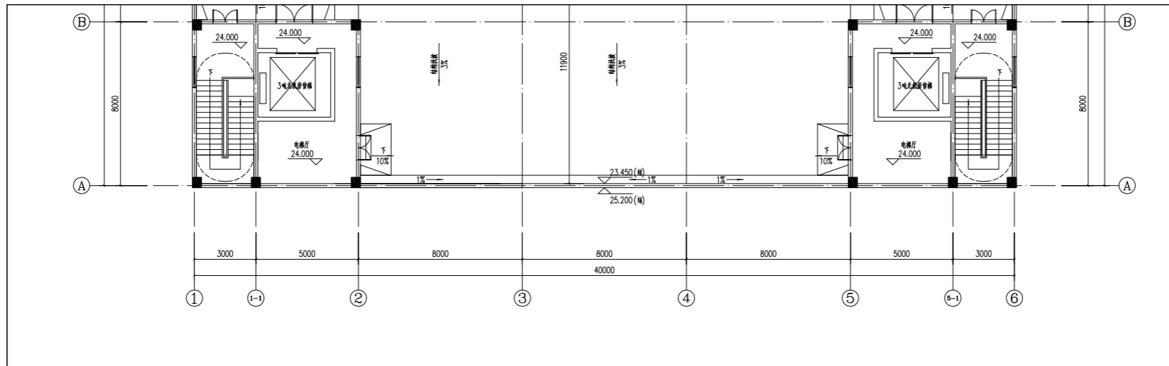
B38#屋面层平面图 1:100
