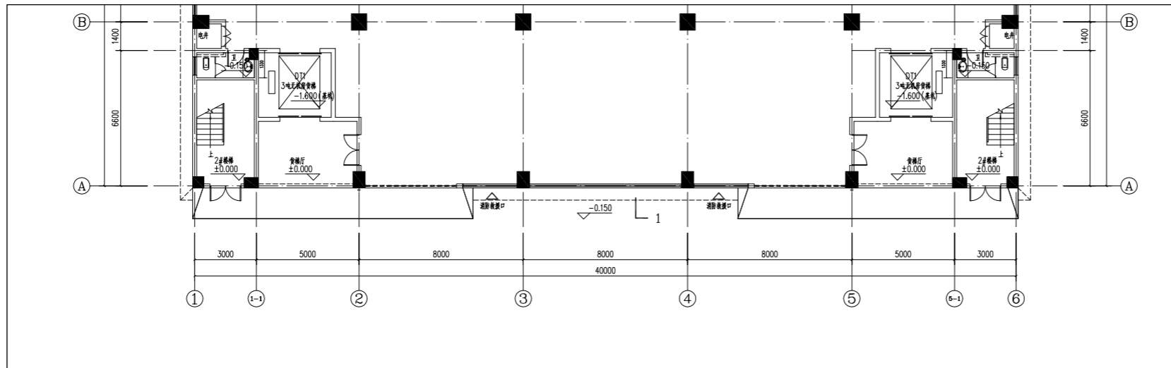
B55#一层平面图 1:100
