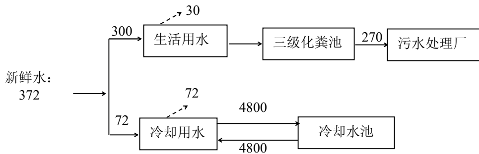
图 2-1 全厂用排水平衡图 (单位: m^3/a )
