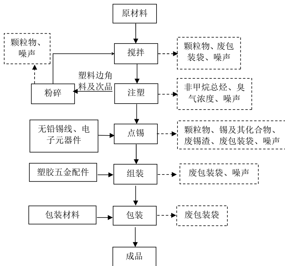
图 2-2 工艺流程图
