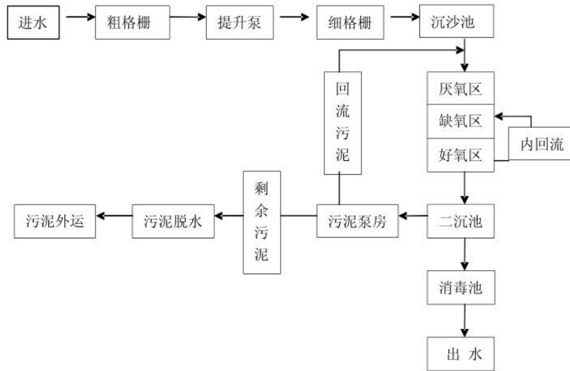
图 4-1 揭阳市区污水处理厂工艺流程图
