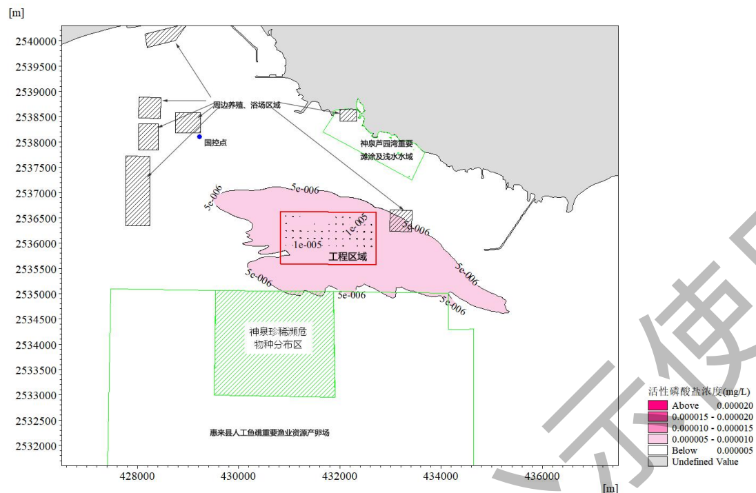
图 5.3.2-6 饵料散失进入海水释放活性磷酸盐浓度增量包络范围
