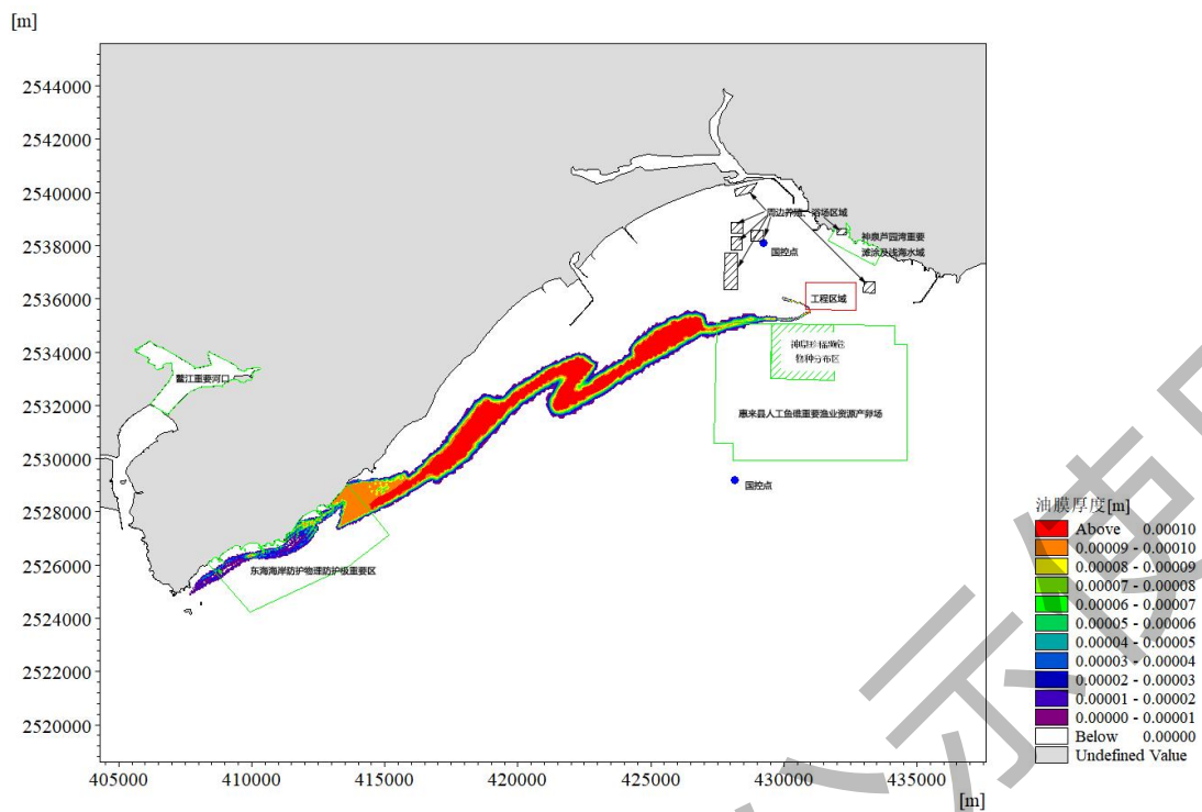
图 6.5.4-1 工况 1 条件下（ENE-3.3m/s，涨初）溢油发生后 72 小时扫海范围
