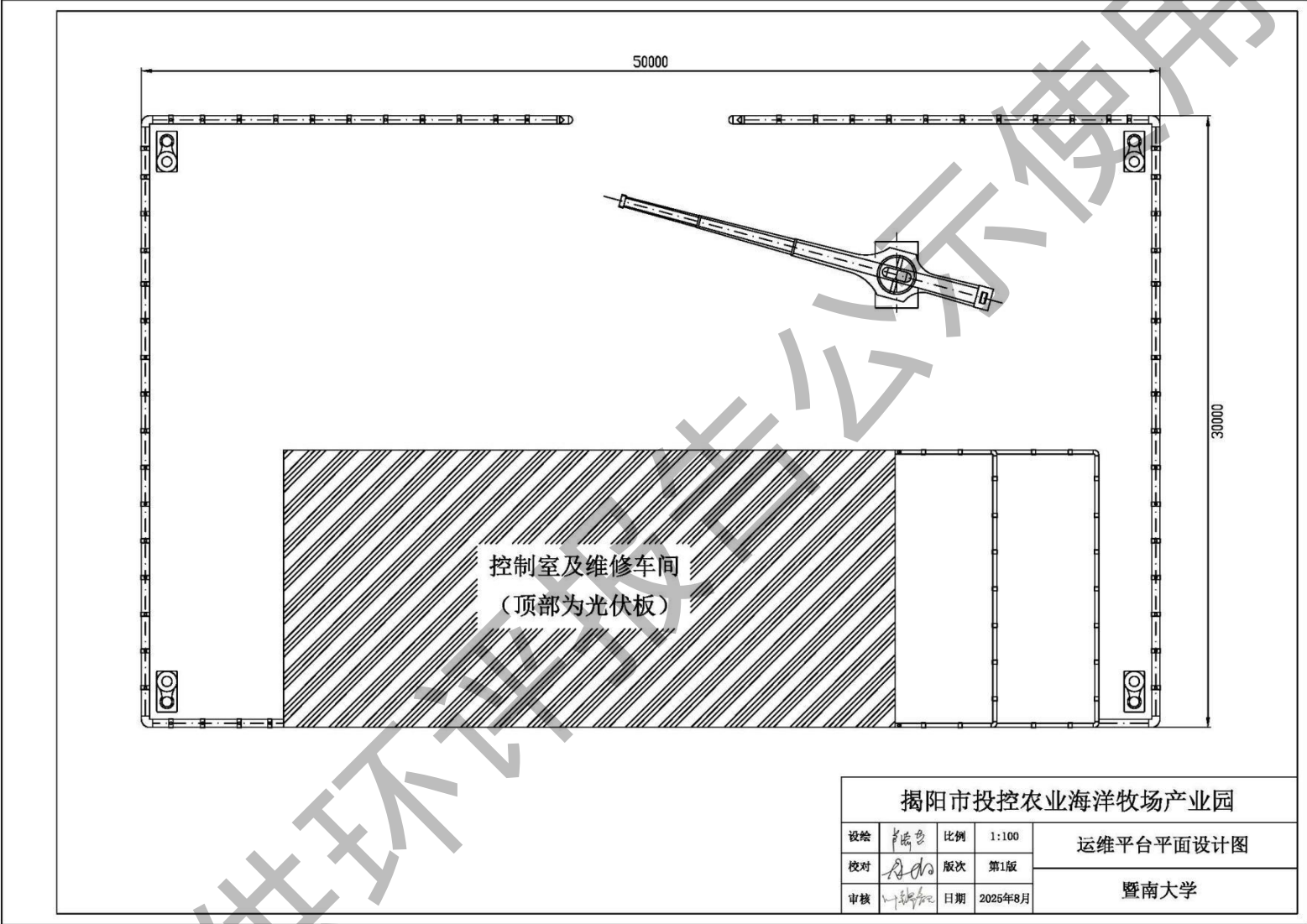
图 3.1.3-4 运维平台平面设计图
