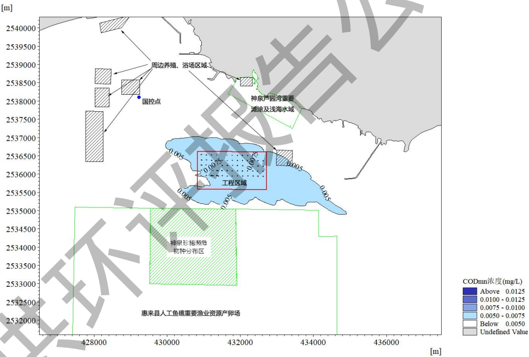
图 5.3.2-1 养殖污染物 COD Mn 浓度增量包络范围
