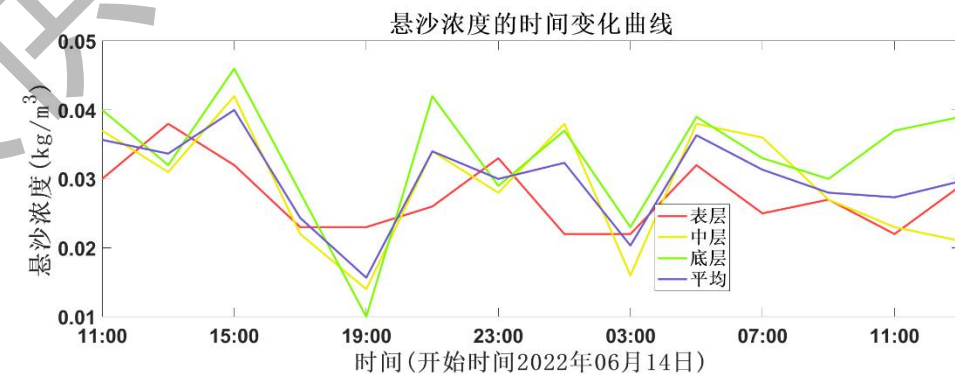
图 4.4.8-6 HLL6 站悬沙浓度时间过程曲线图
