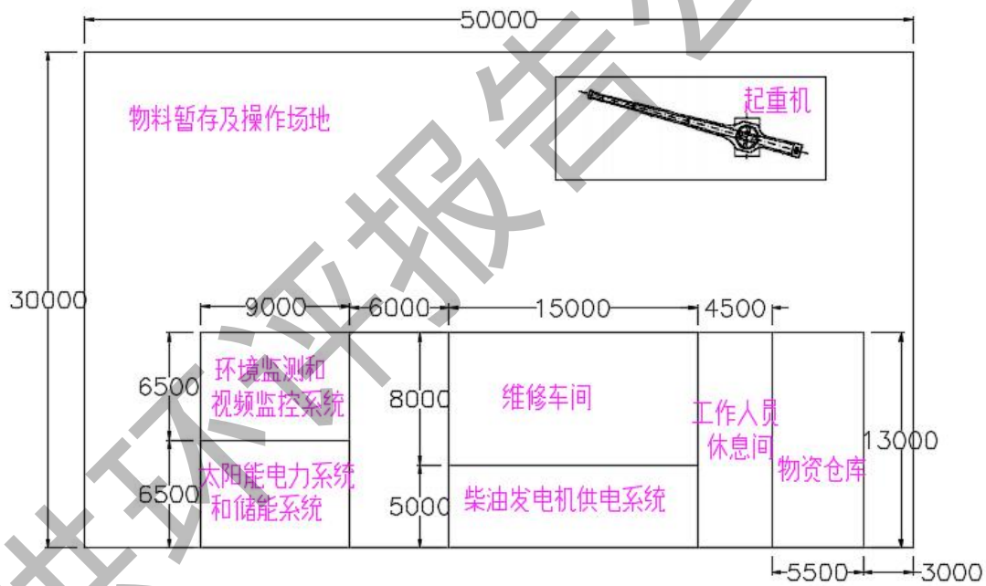
图 3.1.3-8 运维平台功能及布局示意图
