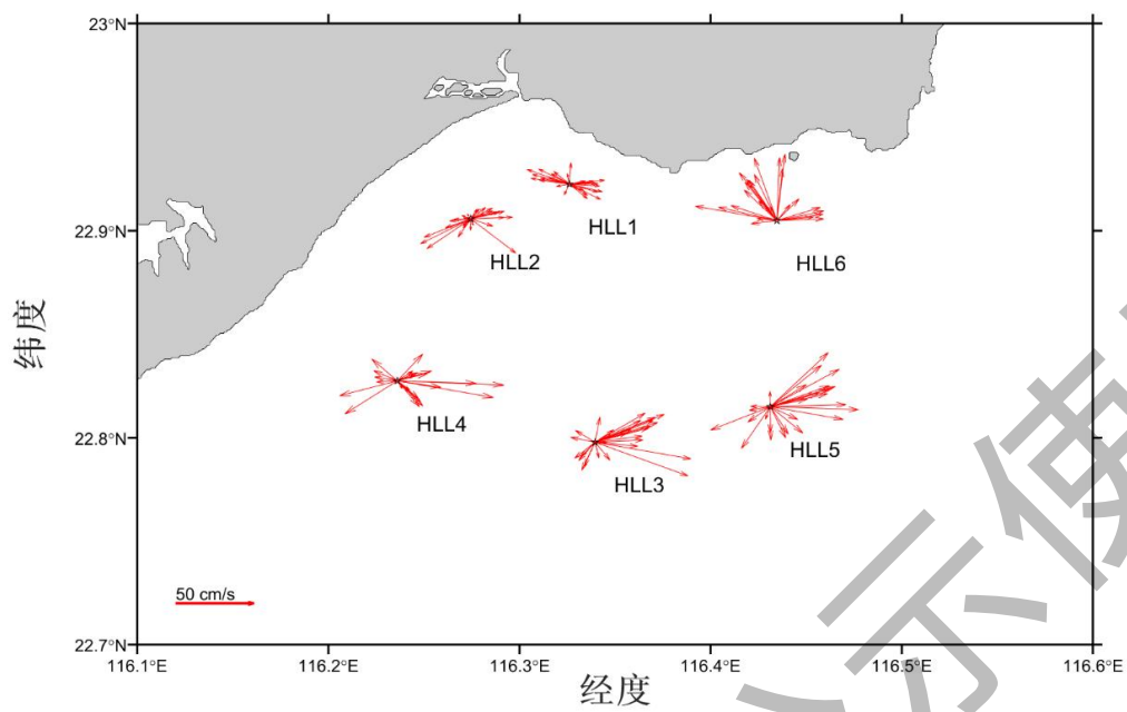
图 4.4.4-2 0.2H 层海流平面分布矢量图
