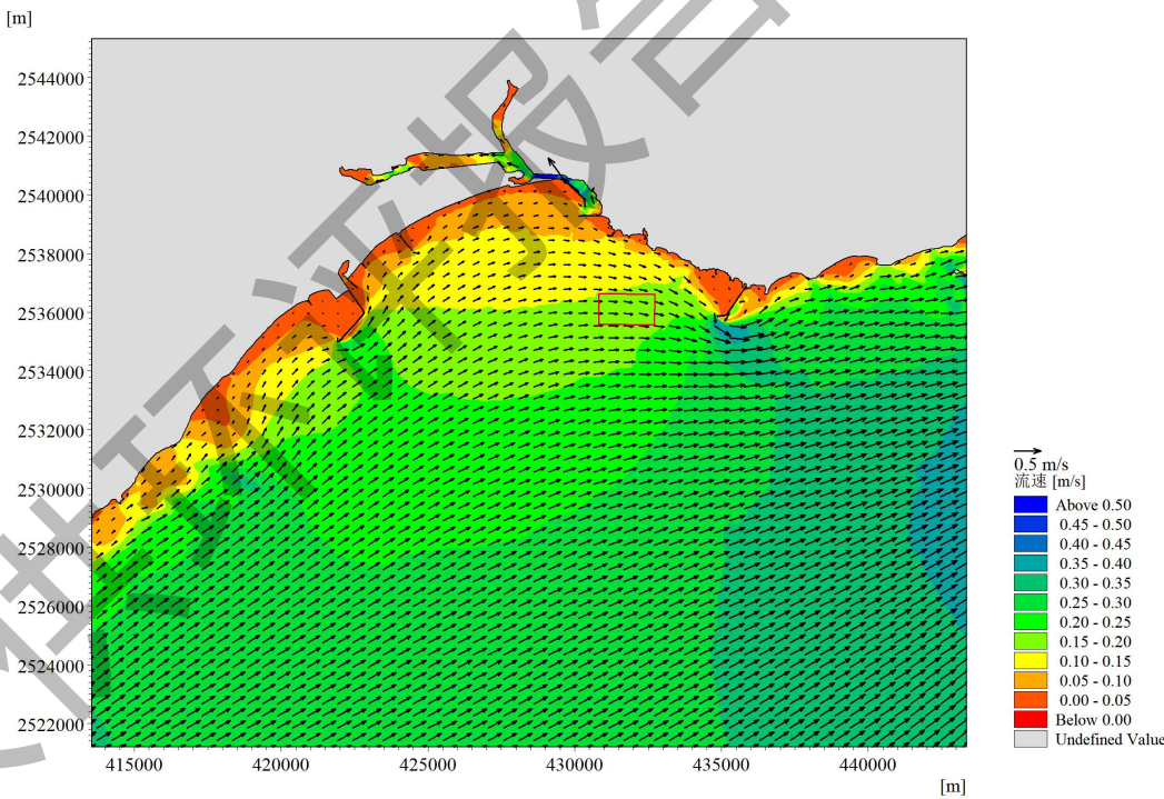
图 5.1.2-1 神泉湾附近大范围海域大潮涨急时刻流场图
