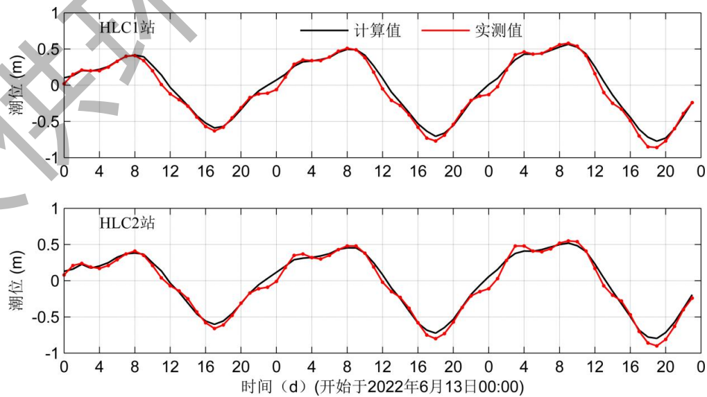
图 5.1.1-5 HLC1、HLC2 站位潮位验证过程线图
