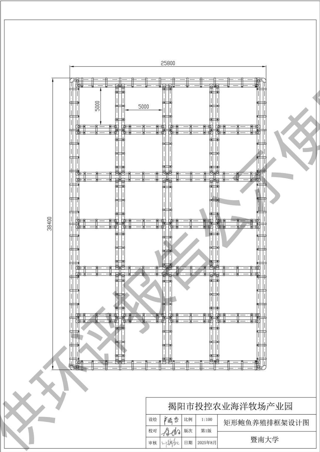
图 3.1.3-3 单个矩形网箱（含 24 个 5 m×5 m 分隔）设计图
