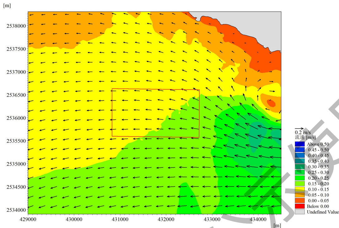
图 5.1.2-4 工程区附近局部海域大潮落急时刻流场图
