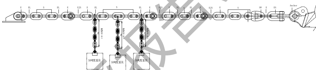
图 3.1.3-9b 锚链配套示意
