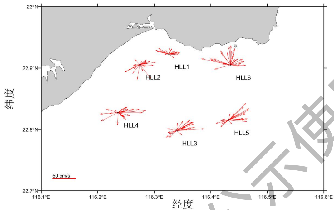
图 4.4.4-4 0.6H 层海流平面分布矢量图
