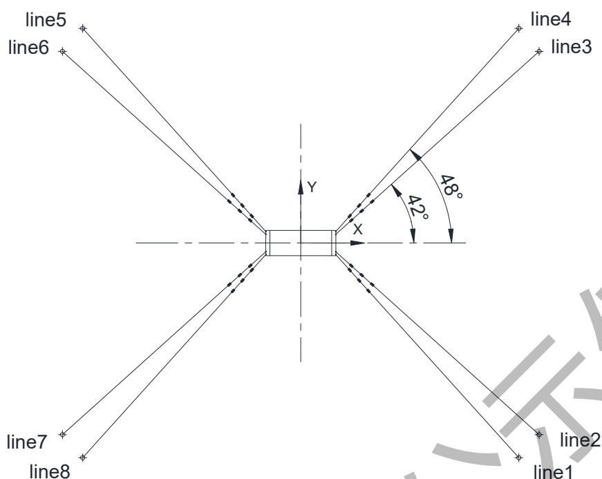
图 3.1.3-9a 锚布置角度
