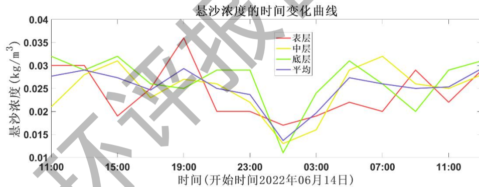
图 4.4.8-5 HLL5 站悬沙浓度时间过程曲线图
