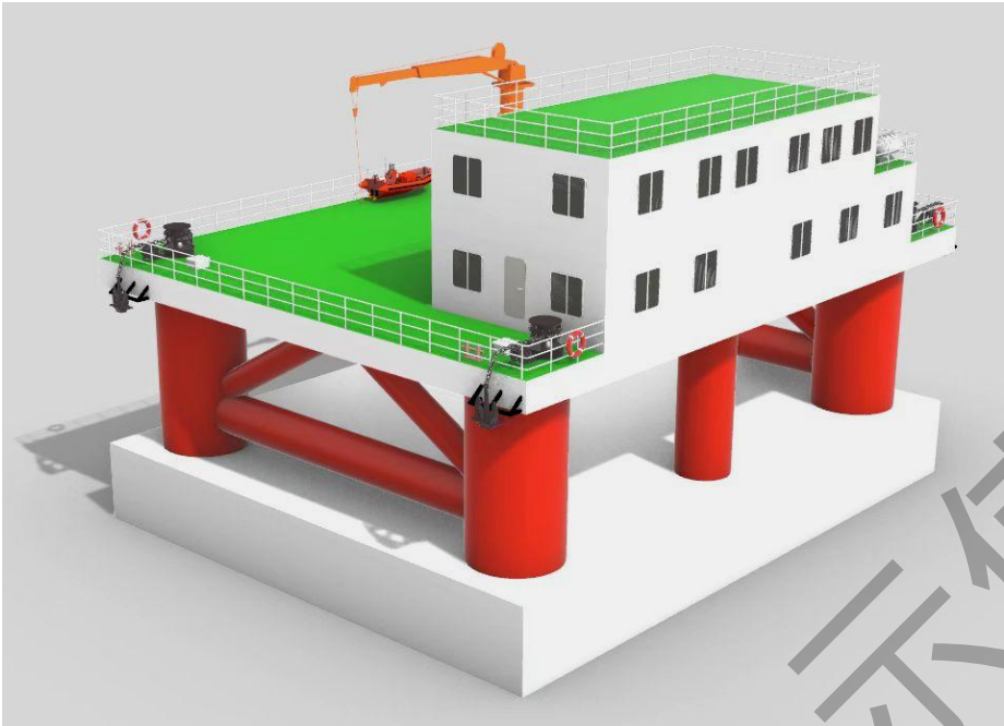
图 3.1.3-7 运维平台示意图
