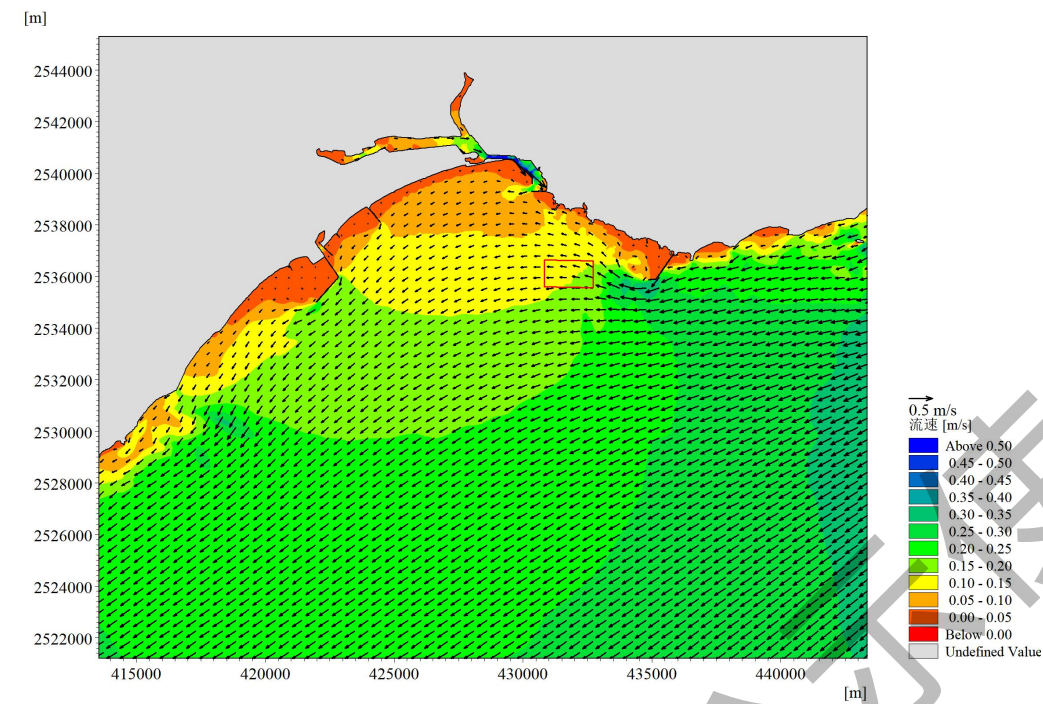
图 5.1.2-2 神泉湾附近大范围海域大潮落急时刻流场图
