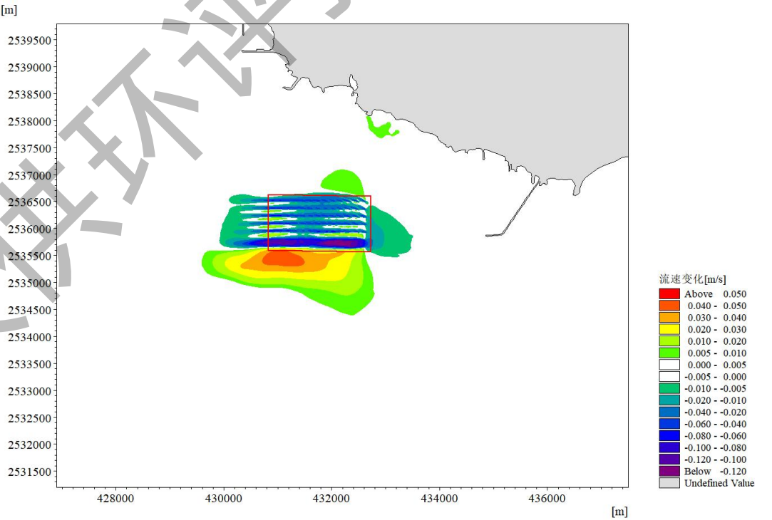
图 5.1.2-6 工程附近海域工程前后大潮落急流速变化等值线图
