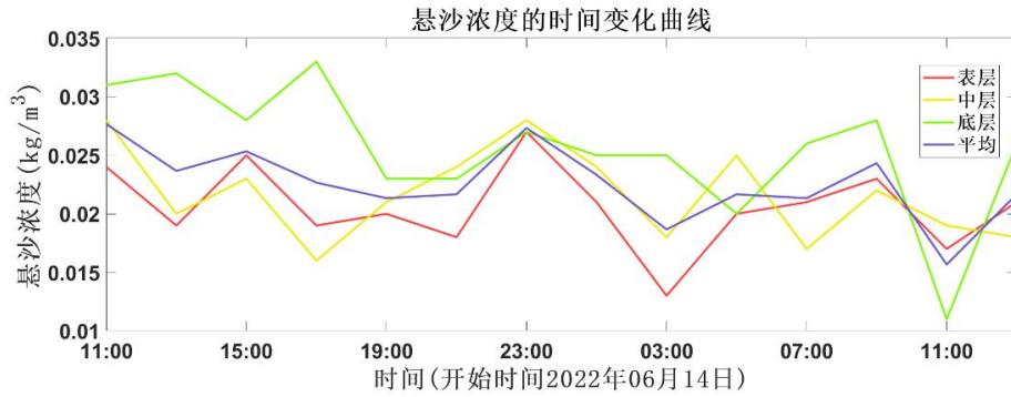
图 4.4.8-3 HLL3 站悬沙浓度时间过程曲线图
