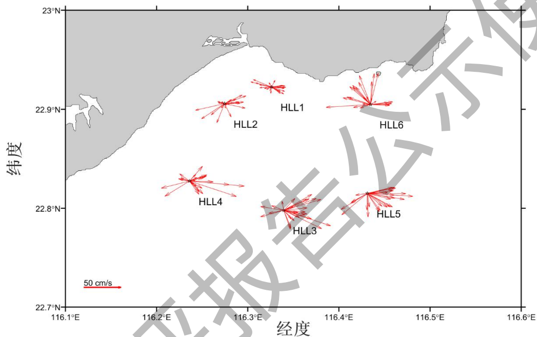
图 4.4.4-1 表层海流平面分布矢量图
