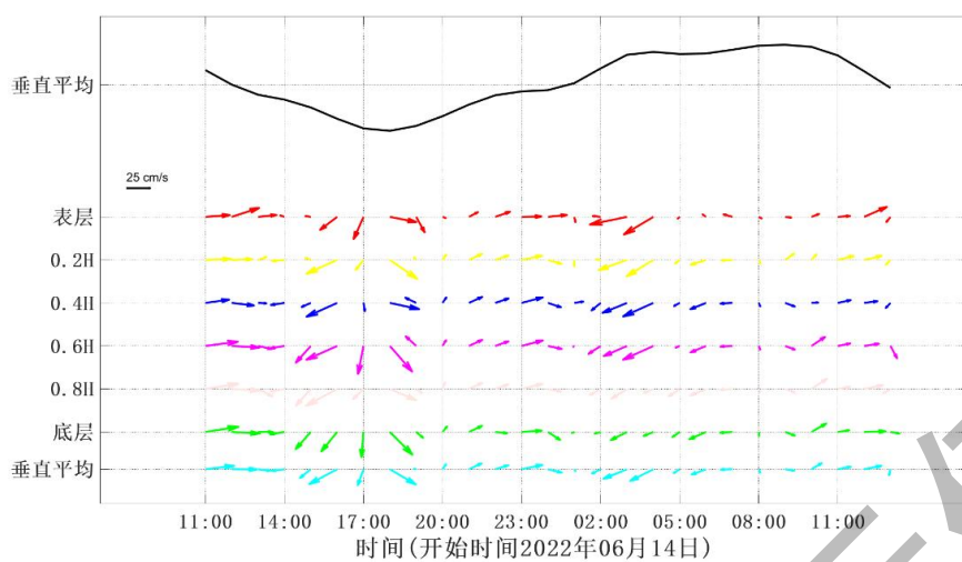
图 4.4.4-8 HLL2 站海流矢量图
