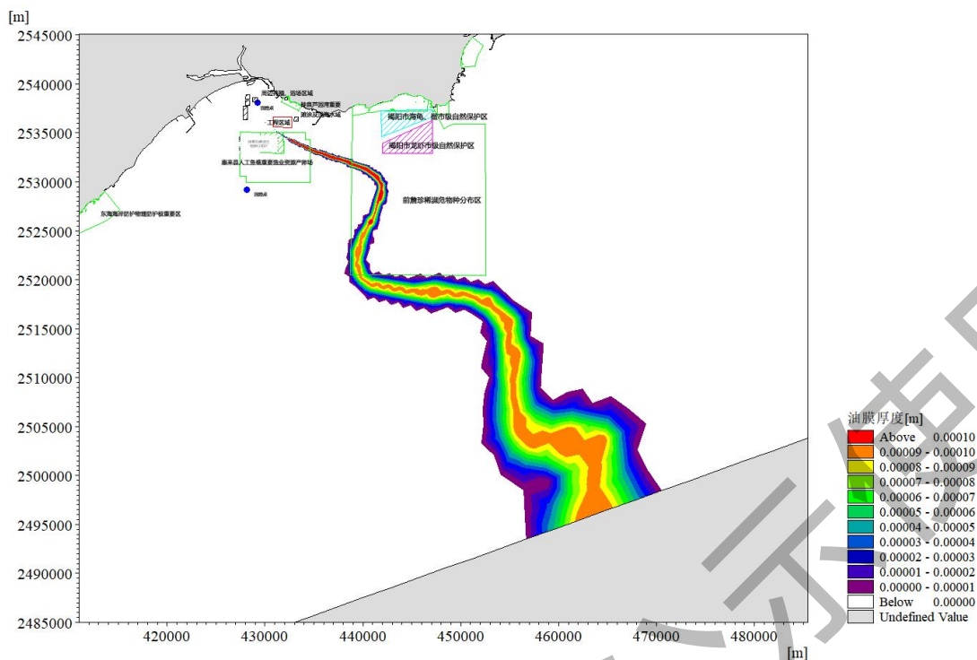
图 6.5.4-5 工况 5 条件下（NW-13.8m/s，涨初）溢油发生后 72 小时扫海范围
