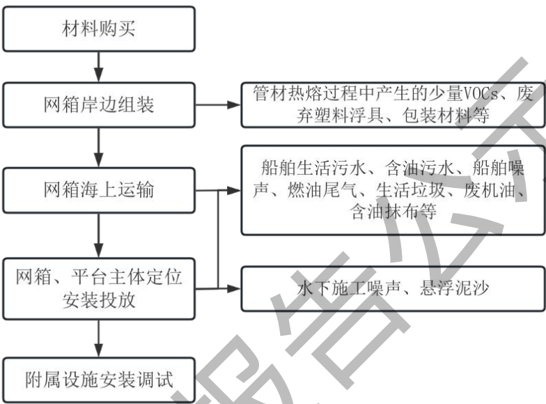
图 3.2.1-1 养殖网箱的施工工艺及产污环节
