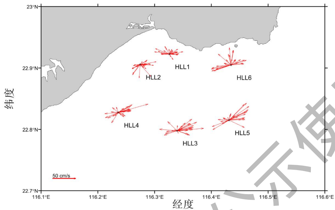
图 4.4.4-6 底层海流平面分布矢量图
