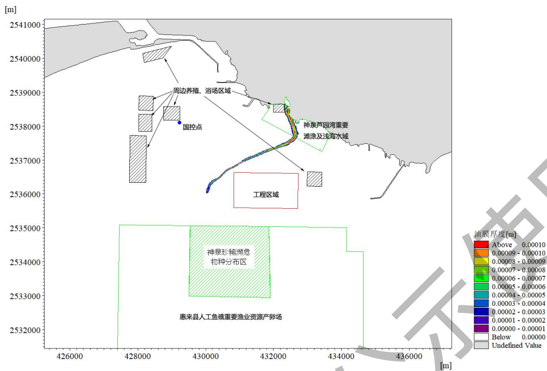
图 6.5.4-3 工况 3 条件下（S-3.4m/s，涨初）溢油发生后 72 小时扫海范围
