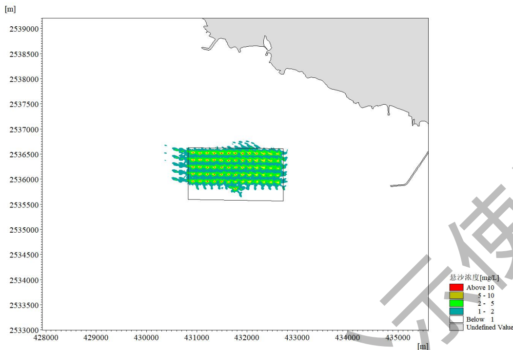
图 5.3.1-3 网箱清洗悬浮物扩散包络范围
