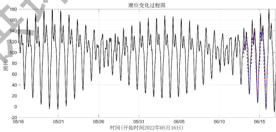
图 4.4.3-4 海门港（广东）潮位过程曲线
