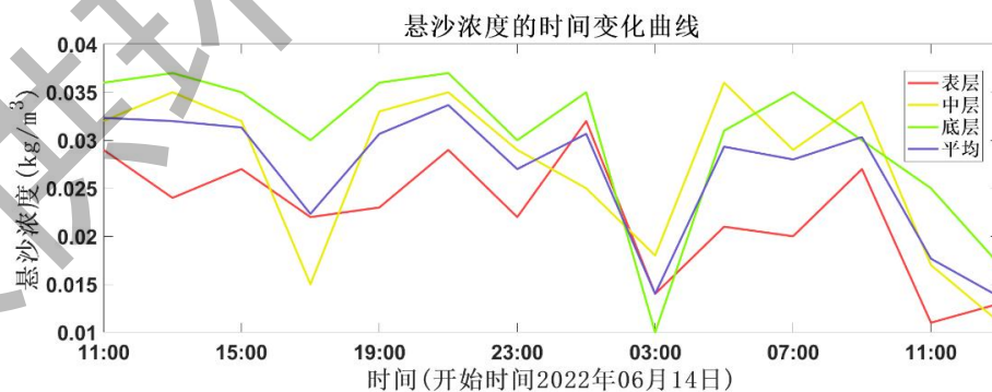
图 4.4.8-2 HLL2 站悬沙浓度时间过程曲线图
