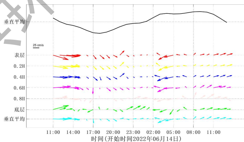
图 4.4.4-10 HLL4 站海流矢量图
