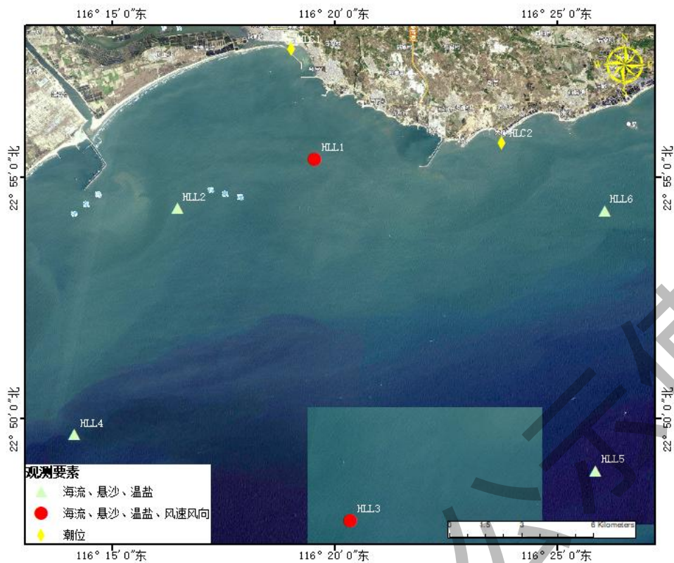
图 5.1.1-4 验证站位布设图
