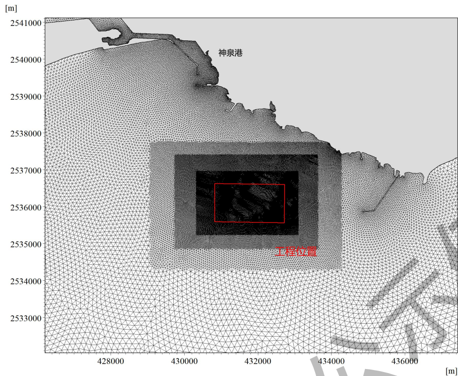
图 5.1.1-2 模型计算网格示意图（工程区附近海域）
