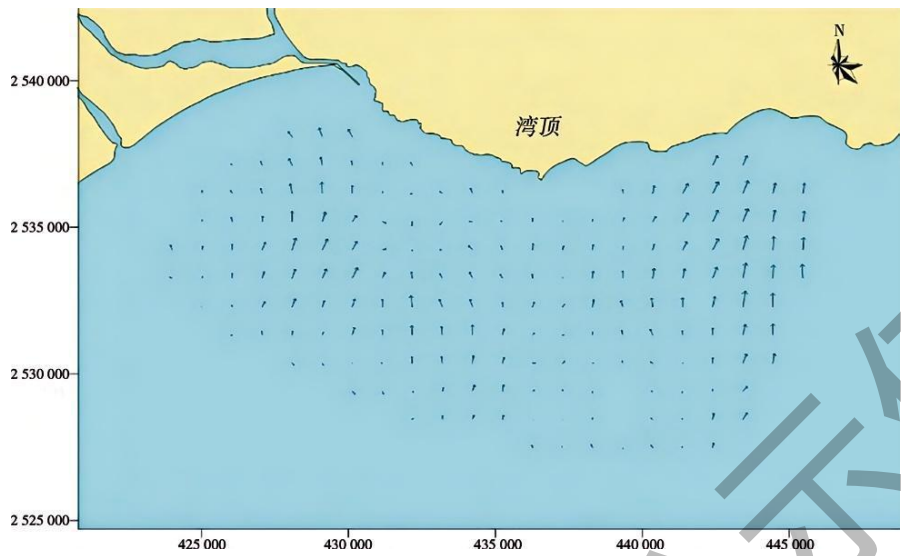
图 4.6.3-2 海域泥沙输运趋势示意图
