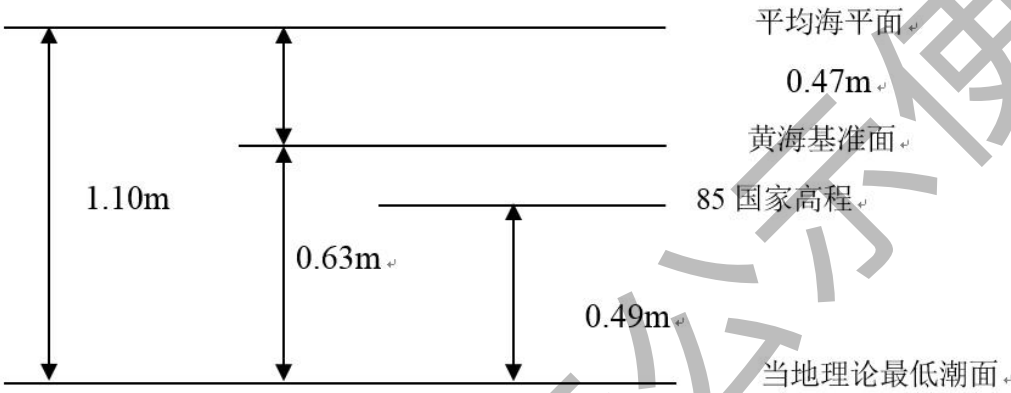
图 4.1.3-1 基面关系图
