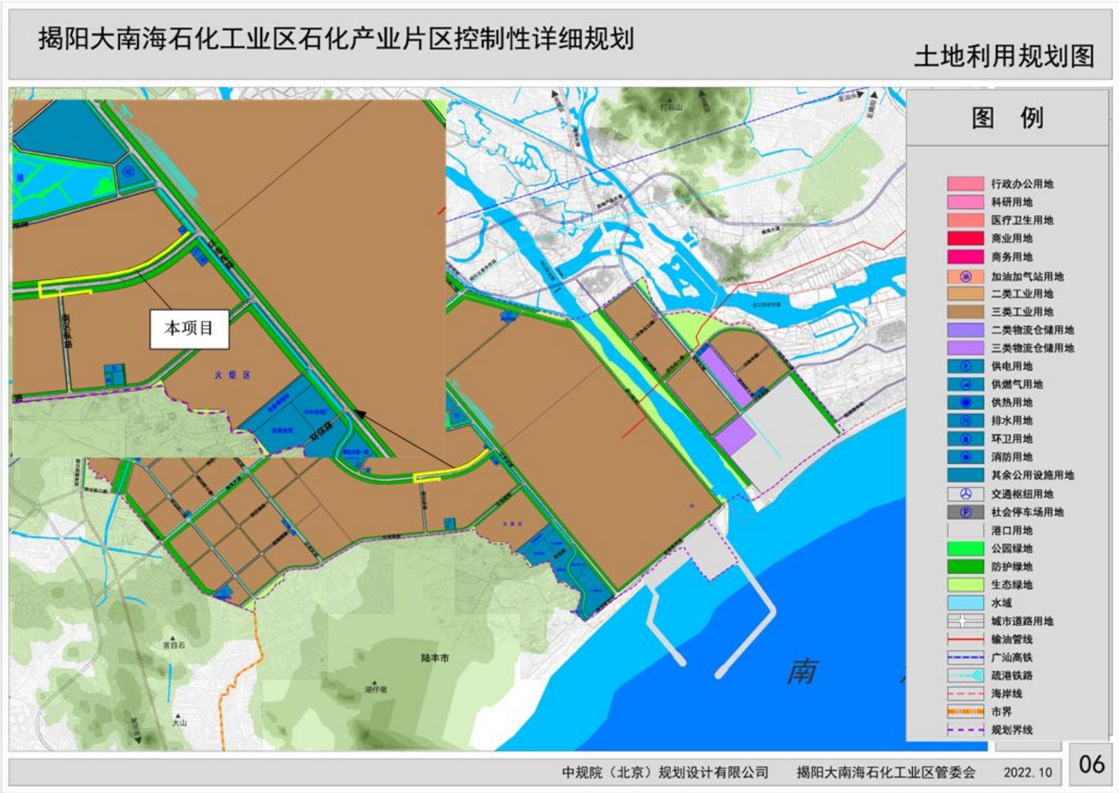
附图 9 揭阳大南海石化工业区石化产业片区控制性详细规划-土地用地规划图
