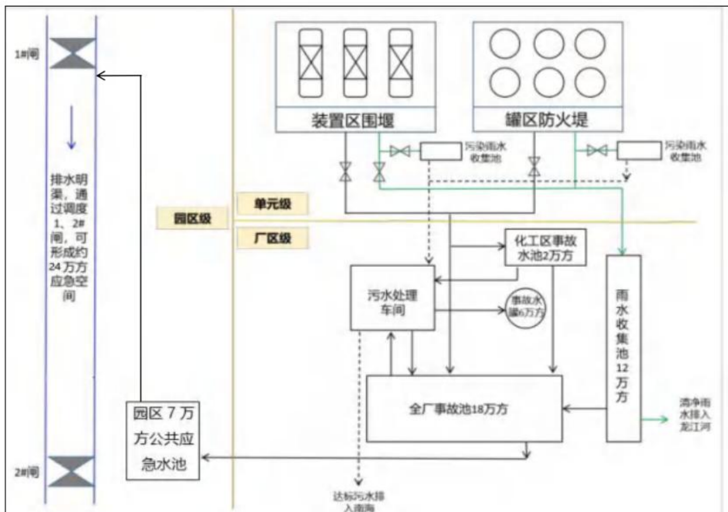
图 5.2-1 广东石化厂区事故水环境风险三级防控体系
