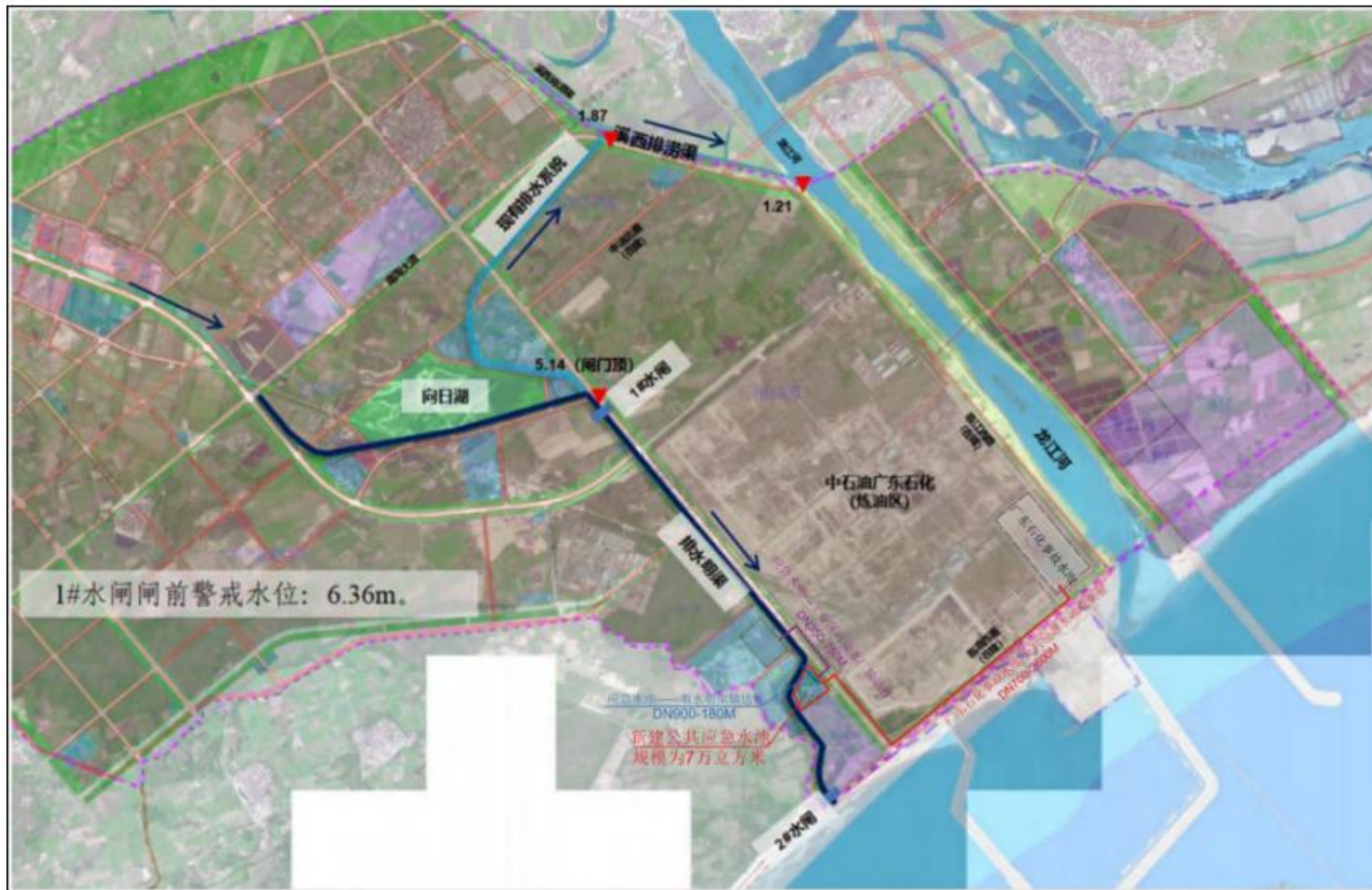
图 5.2-2 大南海石化工业园区公共应急事故水池、西排洪渠以及事故水输送管线情况图
