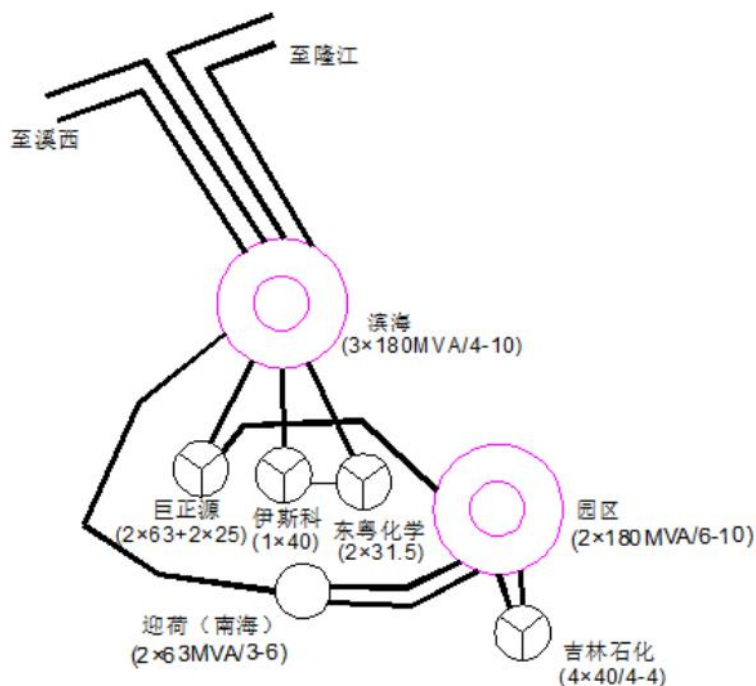
图 2.3-1 110kV 迎荷（南海）站接入系统方案示意图
