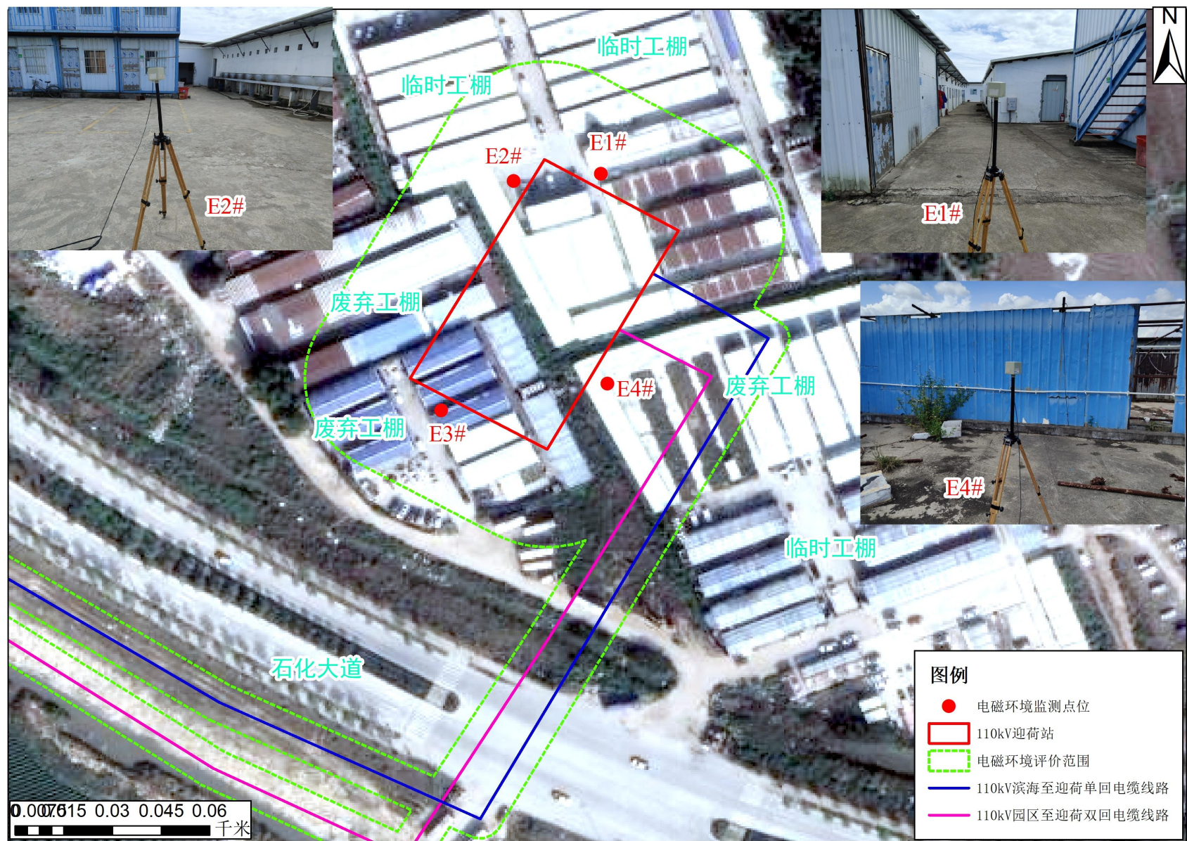
图 8.5-1 电磁监测点位示意图 1
