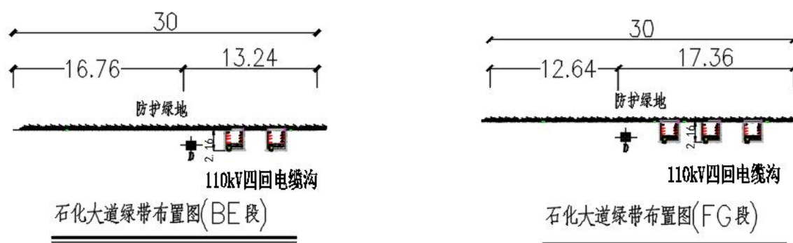
图 2.3-2 石化大道绿带布置图 (BE 段)、(FG 段) 电缆沟断面图
