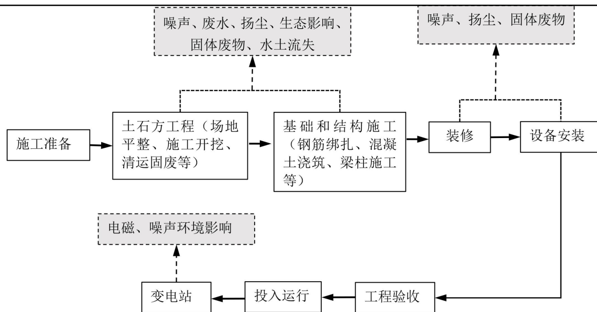
图 2.11-1 变电站施工时序及产污环节图
