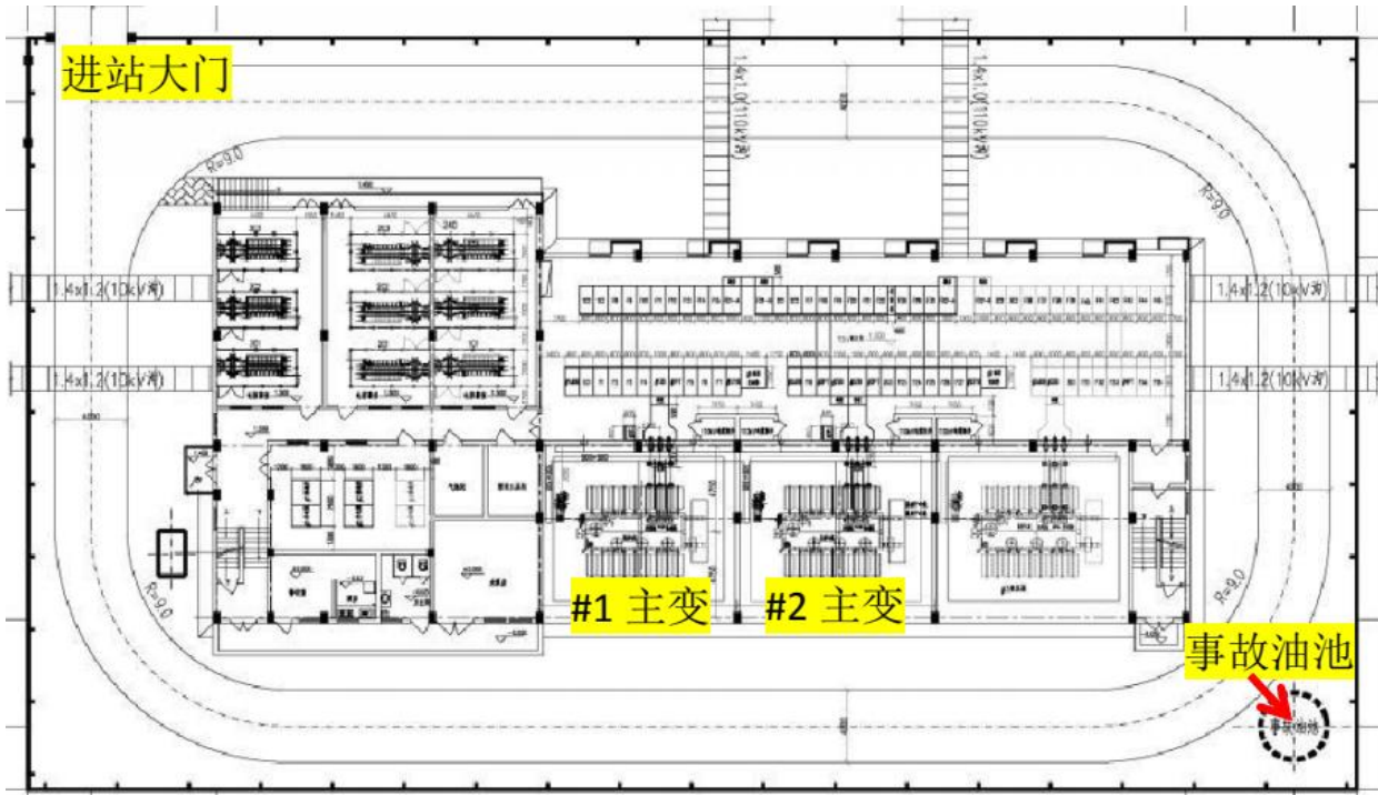
图 9.1-1 惠州 110 千伏曙光变电站总平面布置示意图
