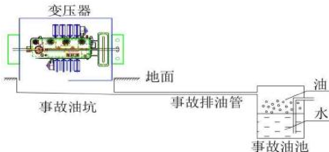
图 2.5-1 事故排油示意图
