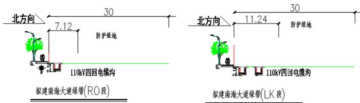
图 2.3-3 拟建南海大道绿带 (RO 段)、(LK 段) 电缆沟断面图
