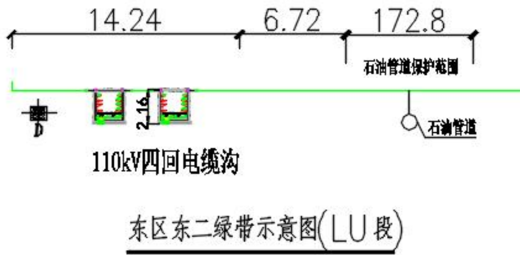
图 2.3-4 东区东二绿带示意图（LU 段）电缆沟断面图
