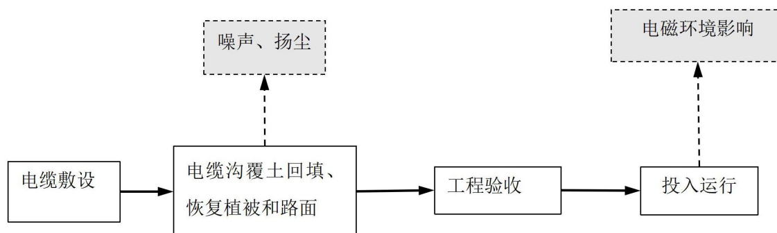
图 2.11-2 电缆线路施工工序流程及产污环节图
