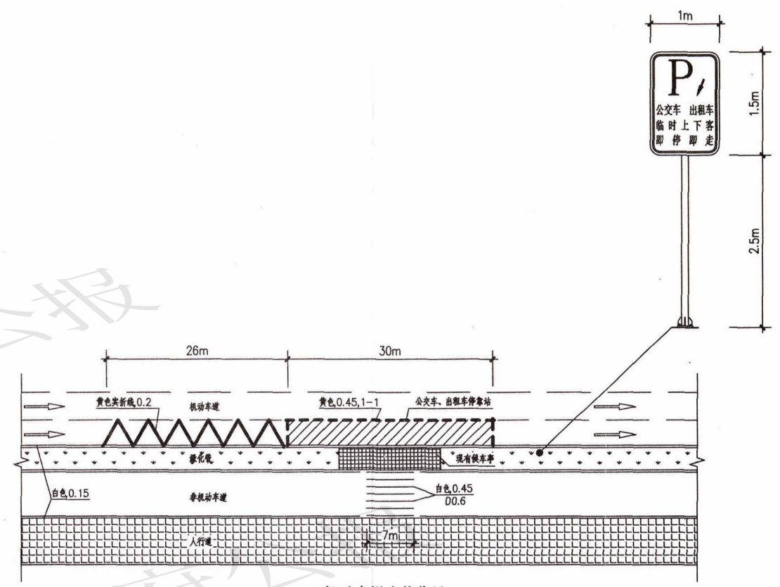
机动车道上停靠站 类型（二）
