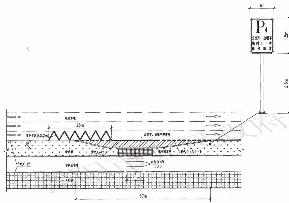
港湾式停靠站 类型（一）
