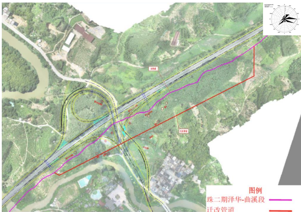
图1.1-2 管道迁改路径图
