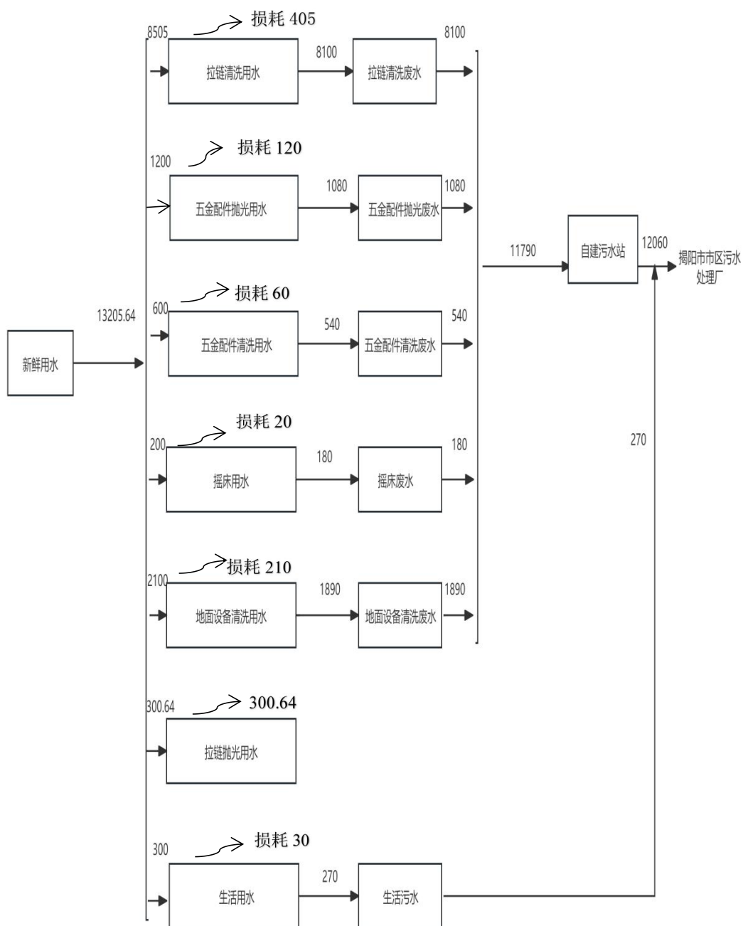
图 2-1 水平衡图 (单位 t/a)
