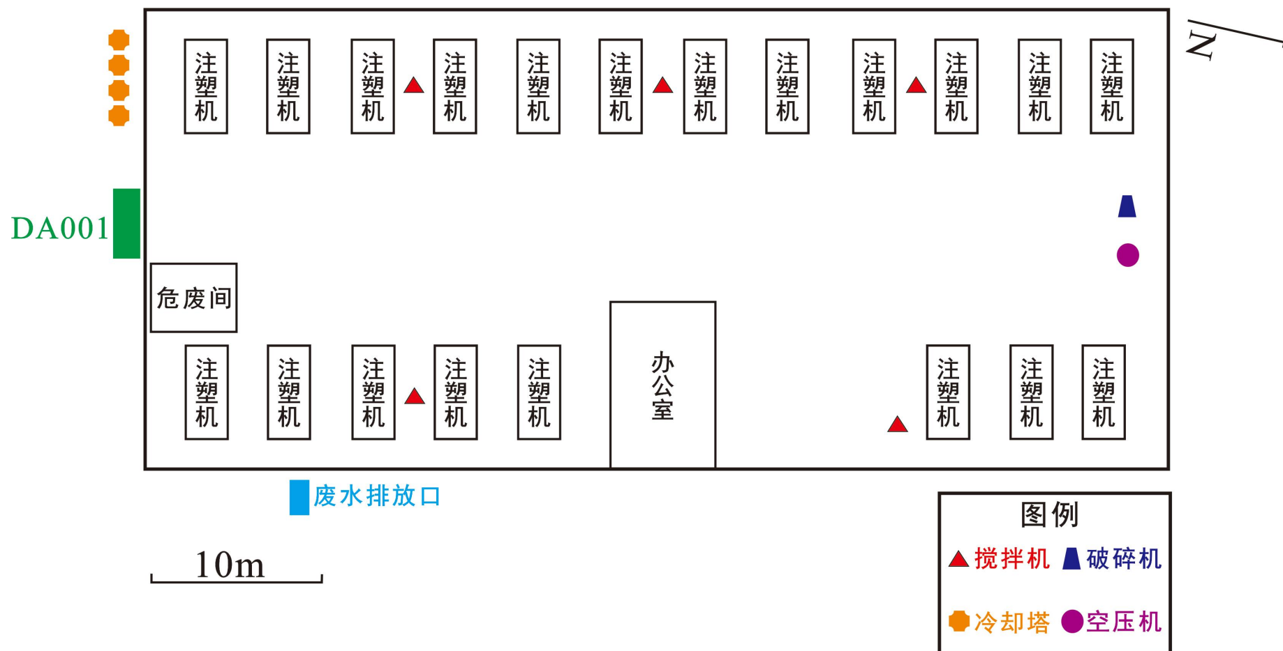
附图 4-1 项目一层平面布置图
