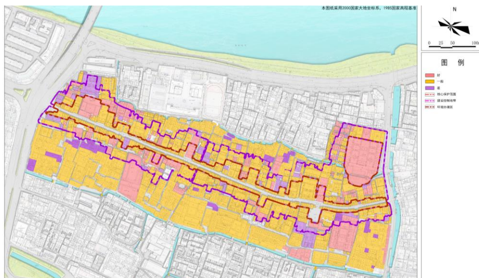
图 4-9 现状建筑质量分析图
