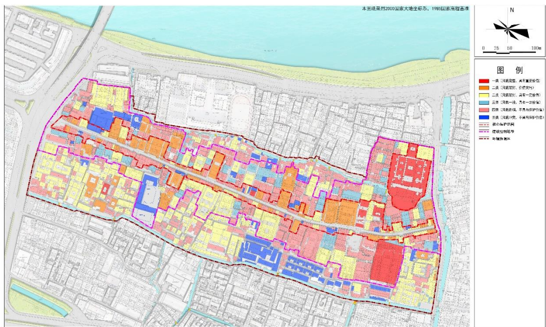
图 4-11 现状建筑风貌分析图
