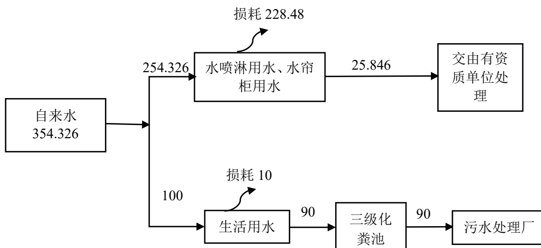
图 1 项目厂区水平衡图 (m³/a)
