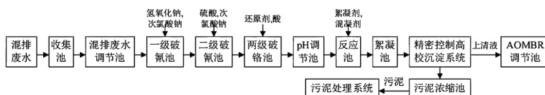
图 7.1-8 混排废水预处理工艺流程图
