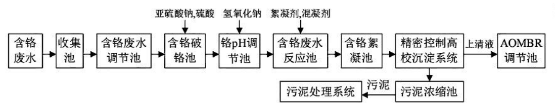
图 7.1-3 含铬废水预处理工艺流程图
