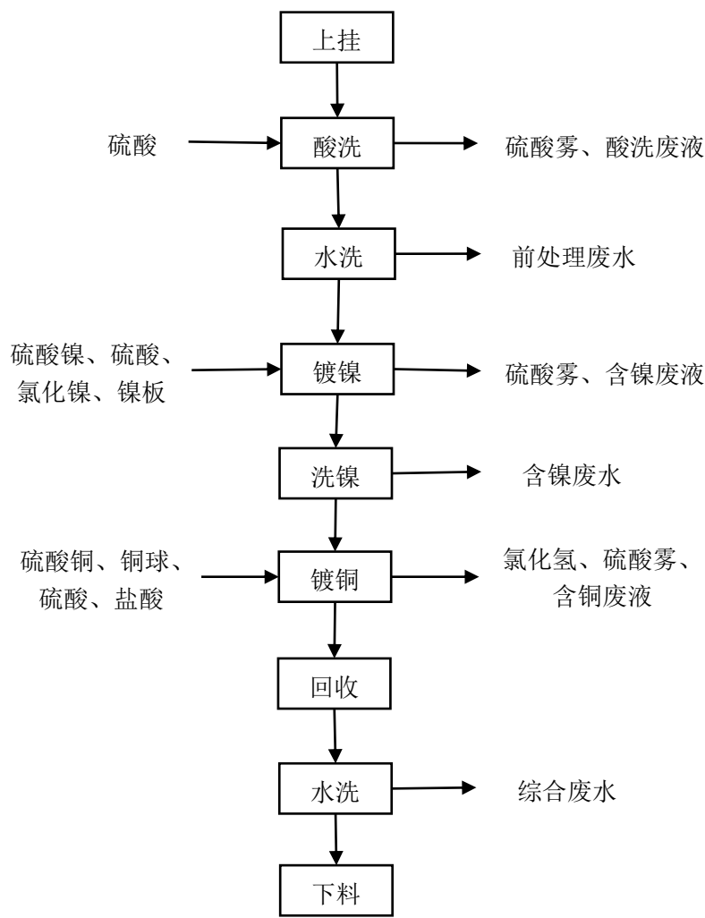
图 4.6-1 项目镀铜镍线生产工艺流程图
