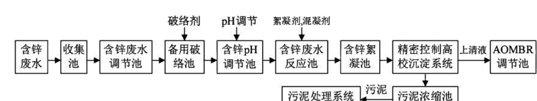
图 7.1-2 含锌废水预处理工艺流程图
