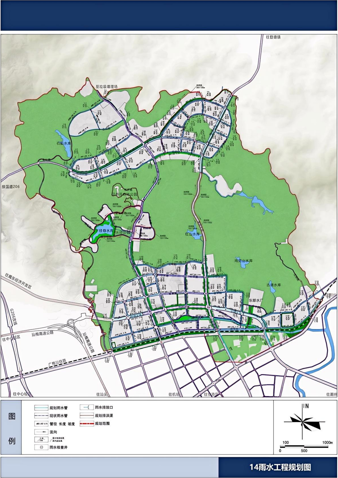
图3.1-5雨水工程规划
