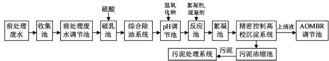
图 7.1-1 前处理废水预处理工艺流程图
