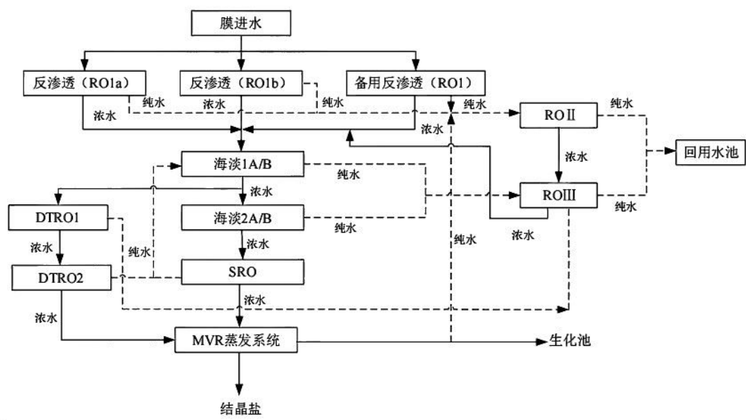
图 7.1-10 膜浓回用处理工艺流程图
