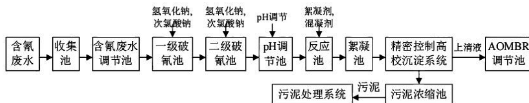
图 7.1-5 含氰废水预处理工艺流程图
