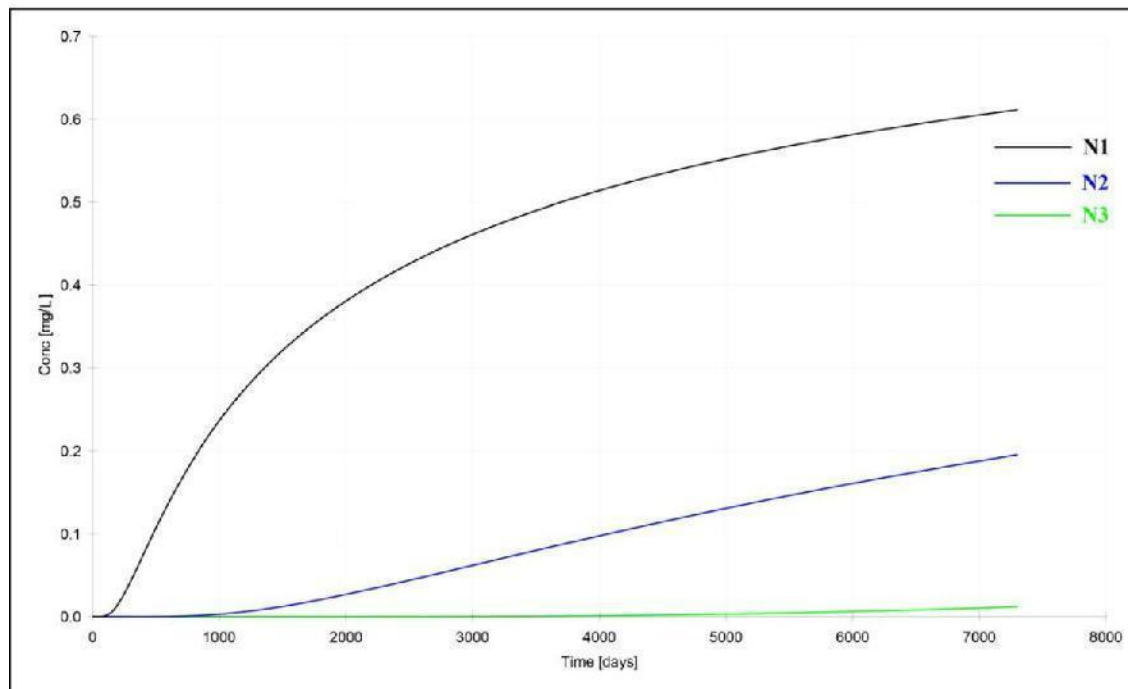
图 6.7-2 pH 浓度-时间曲线
