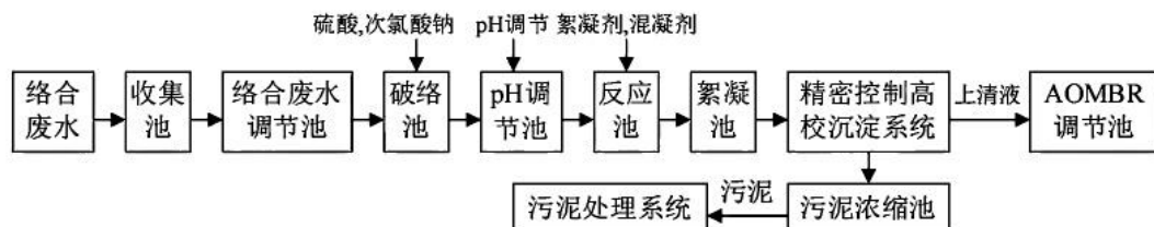
图 7.1-6 络合废水预处理工艺流程图
