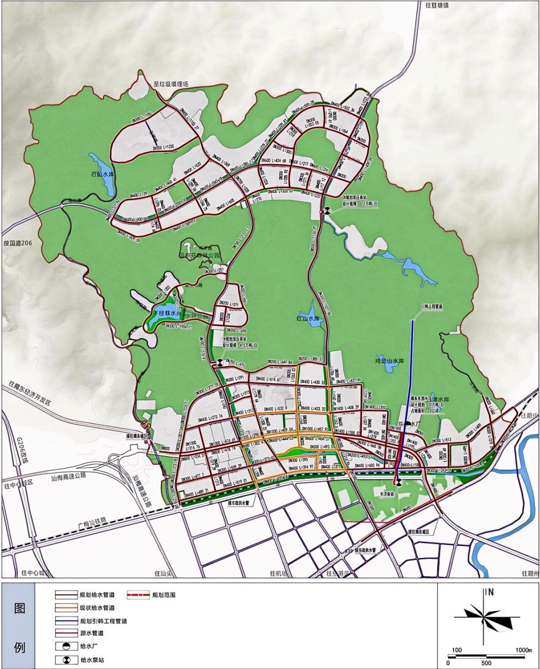
图3.1-4给水工程规划
