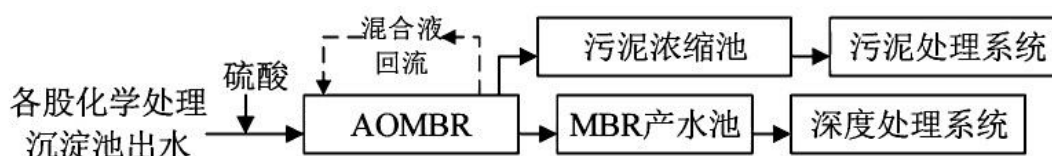
图 7.1-9 生化处理工艺流程图
