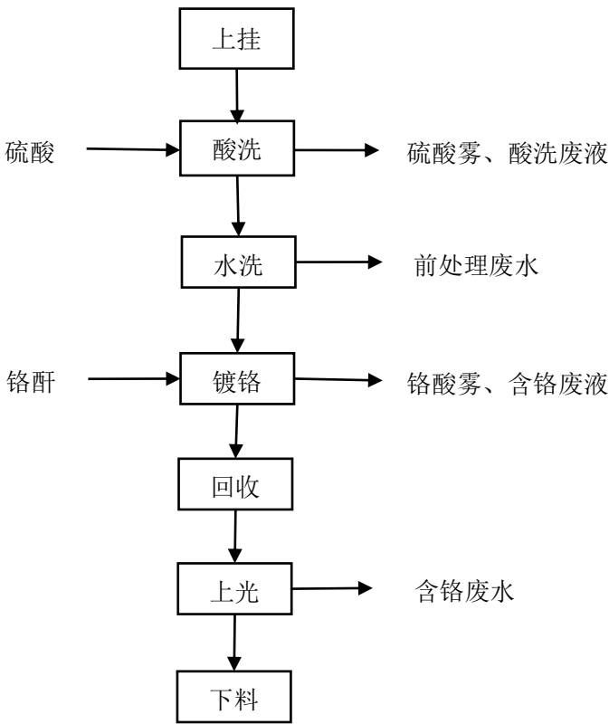
图 4.6-2 项目镀铬线生产工艺流程图
