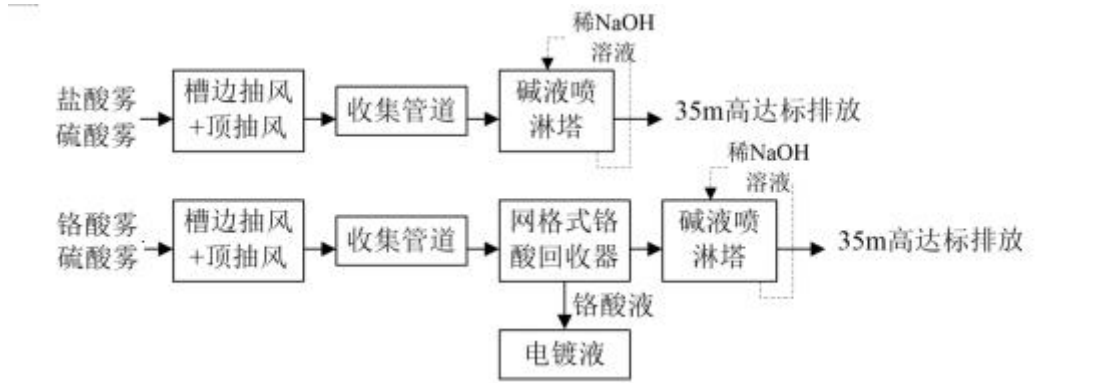
图7.3-1 酸雾废气处理系统工艺流程
