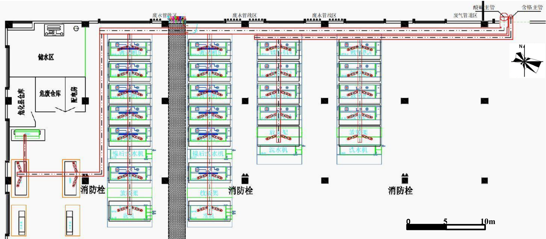
图 4.1-4 项目车间内抽风布管示意图
