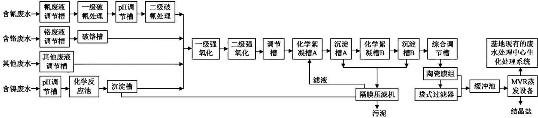
图 7.1-12 高浓废水处理系统工艺流程图
