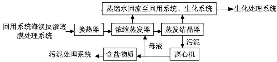
图 7.1-11 MVR 系统处理工艺流程图
