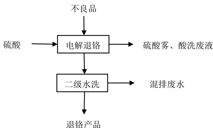
图 4.6-3 项目退铬生产工艺流程图
