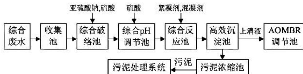
图 7.1-7 综合废水预处理工艺流程图
