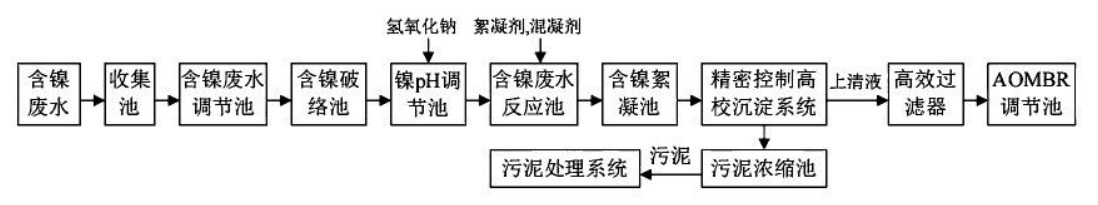
图 7.1-4 含镍废水预处理工艺流程图
