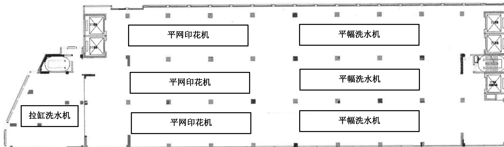
图 3.3-8 原有项目（A 栋厂房）5 楼平面布置图
