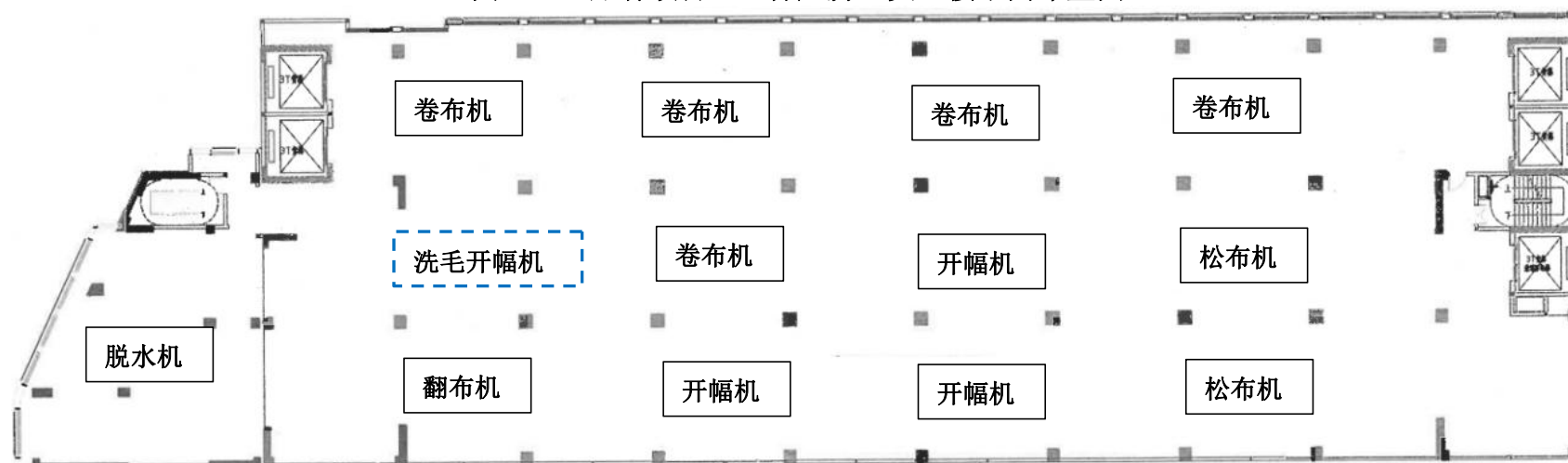
图 3.3-4 原有项目（A 栋厂房）1 楼平面布置图
