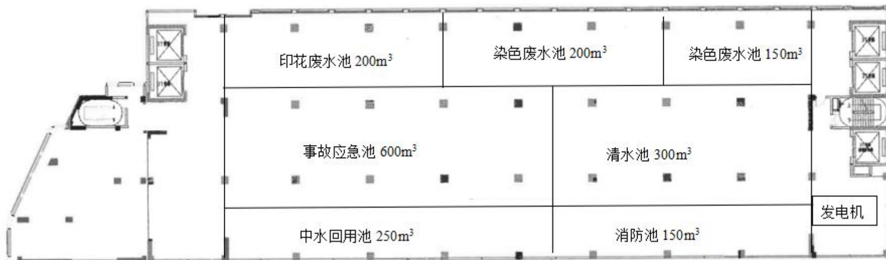
图 4.1-2 本项目厂房负 1 楼平面布置图
