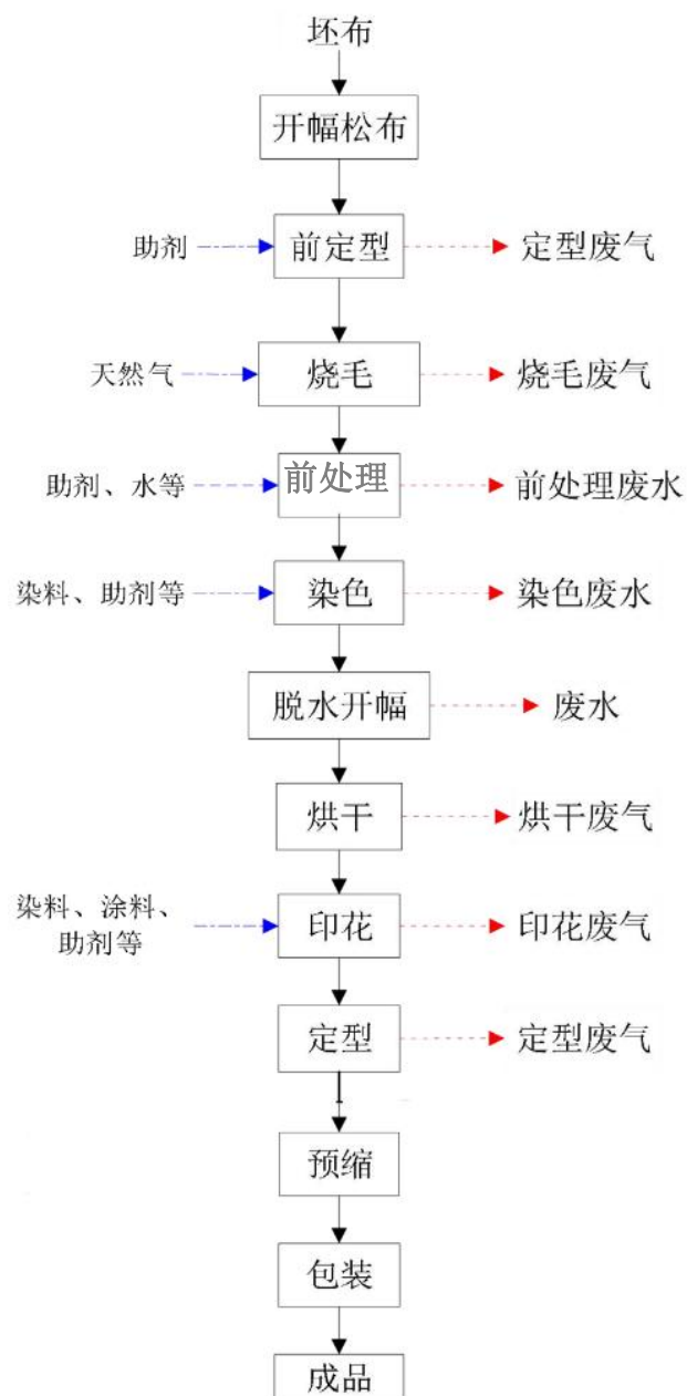
图 4.4-1 坯布染整生产工艺流程图
