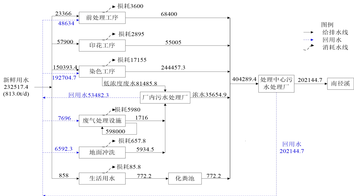
图 3.4-5 原有项目水平衡图 (单位:m 3 /a)
