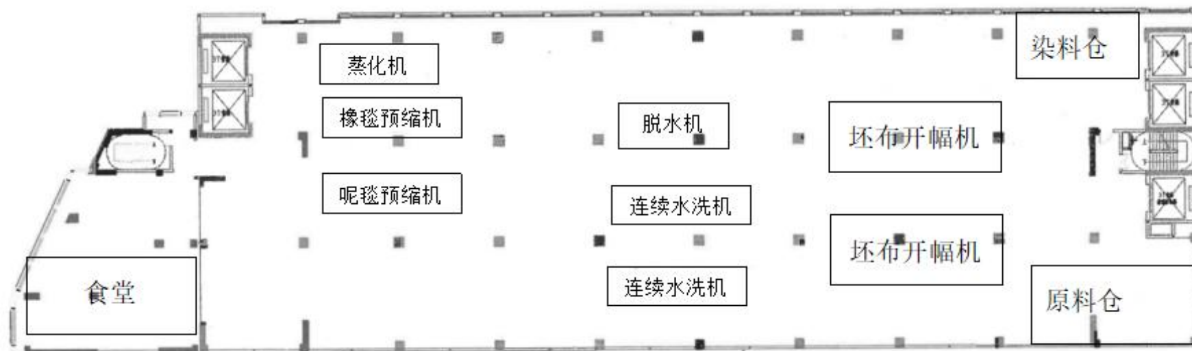
图 4.1-4 本项目厂房 2 楼平面布置图
