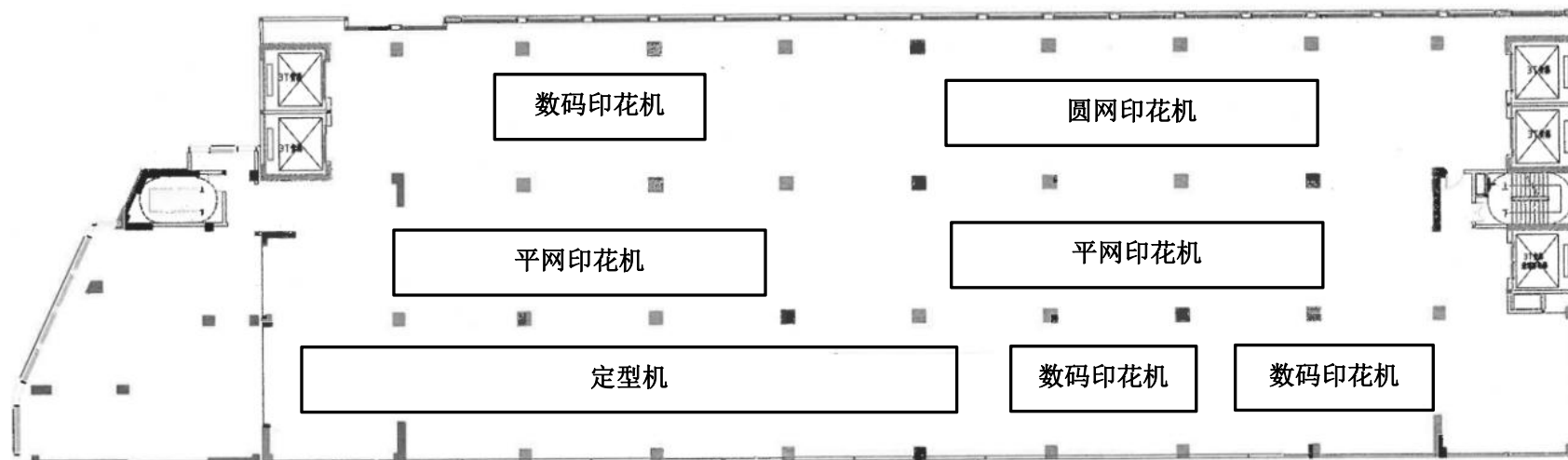
图 3.3-9 原有项目（A 栋厂房）6 楼平面布置图
