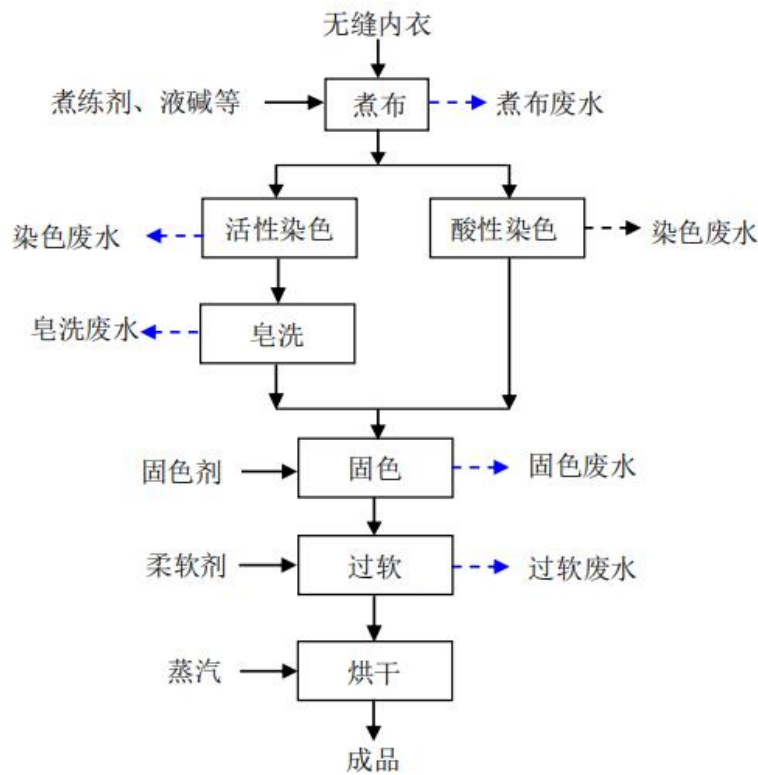
图 4.4-3 无缝内衣染色工艺流程及产污环节图
