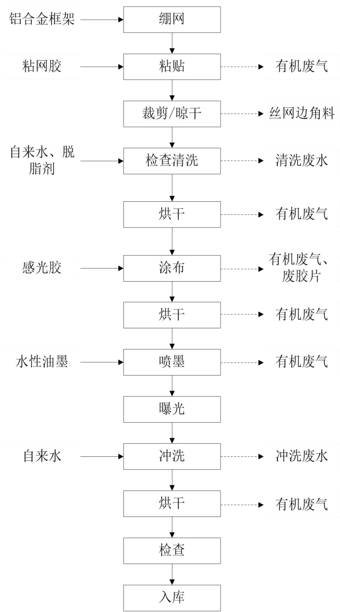
图 4.4-4 印花网版制作工艺流程及产污环节图
