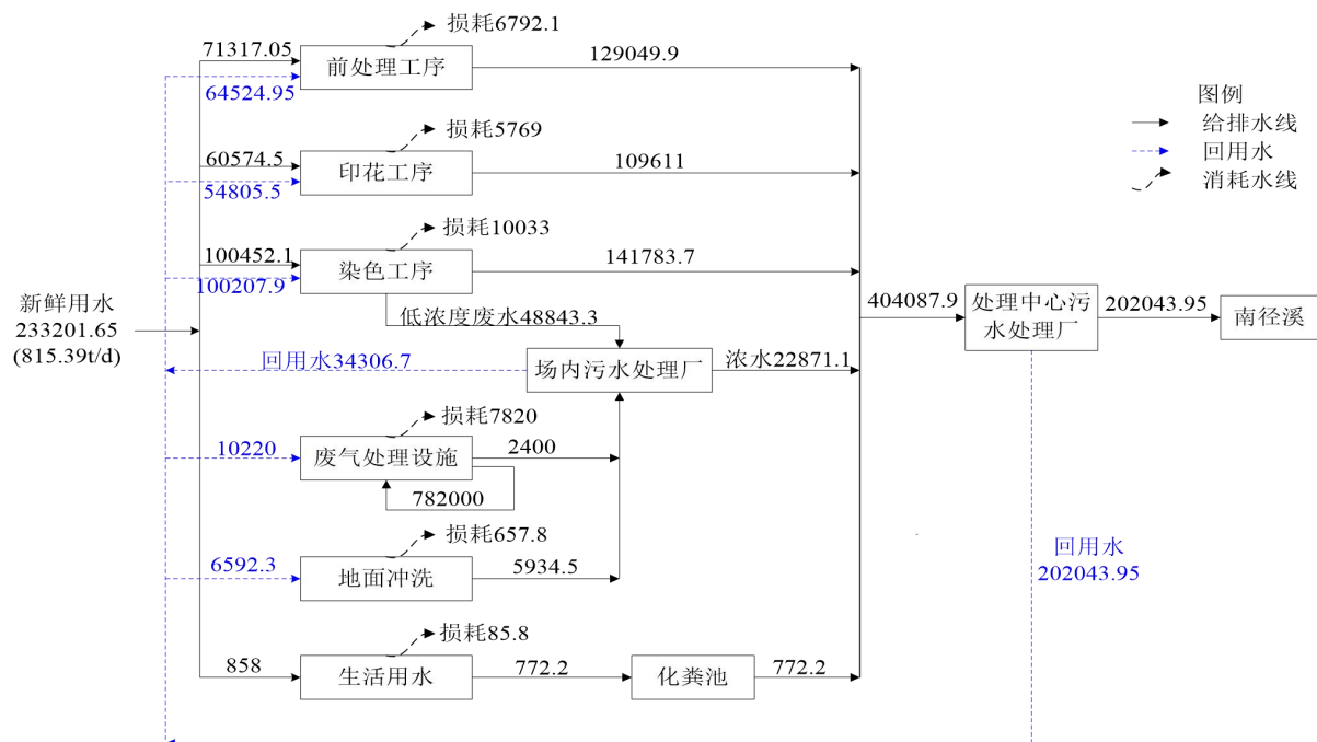
图 4.4-8 项目水平衡图 (单位:m³/a)
