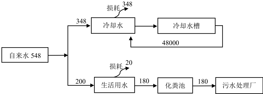
图 2-1 项目用水平衡图 (t/a)
