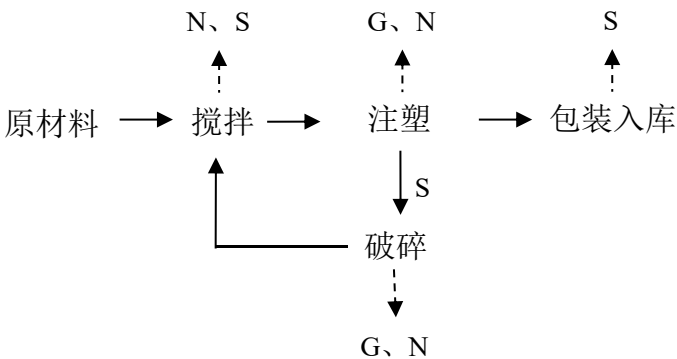
图 2-2 日用塑料制品生产工艺流程图
