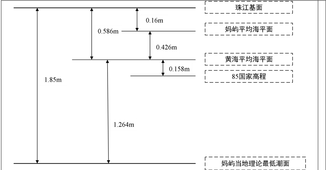
图 2.2.2-1 基面关系图
