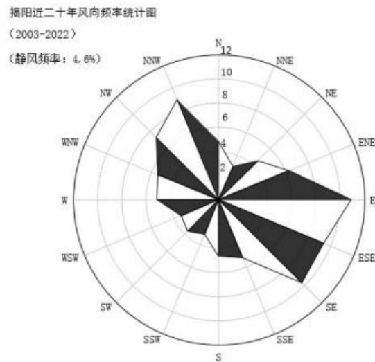
图 2.2.2-1 揭阳气象站风向玫瑰图
