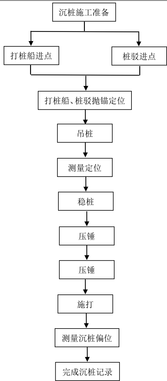
图 1.12-1 钢筋砼预制方桩施工工艺流程图
