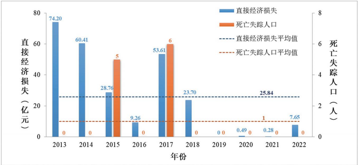
图 2.2.10-1 2013-2020 年广东省风暴潮灾害直接经济损失和死亡失踪人数统计
