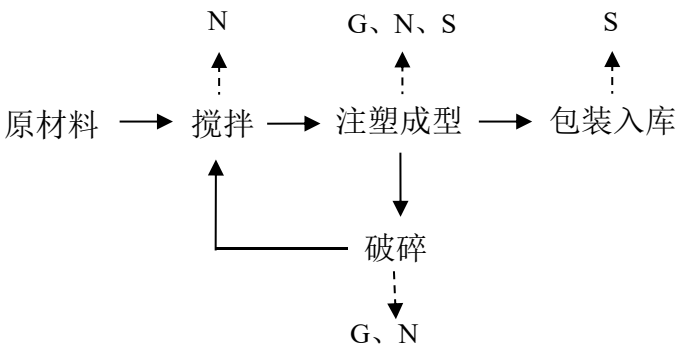
图 2-2 日用塑料制品生产工艺流程图
