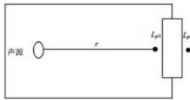
图4-1 室内声源等效为室外声源图例
