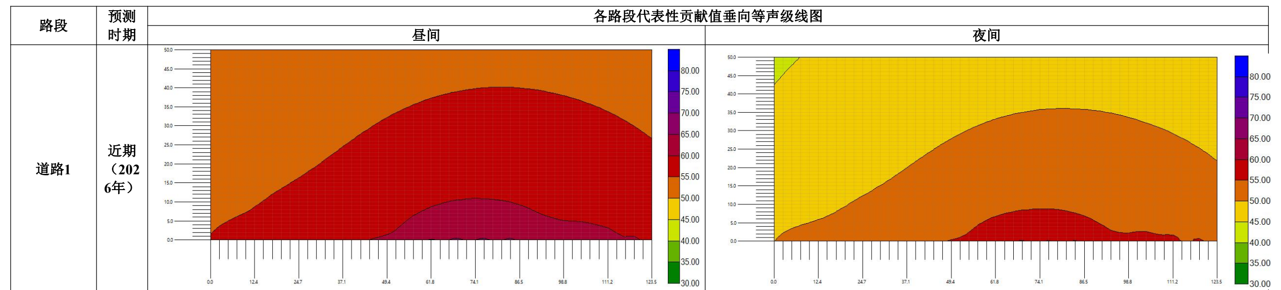
图 16 项目交通噪声预测等声级线图
