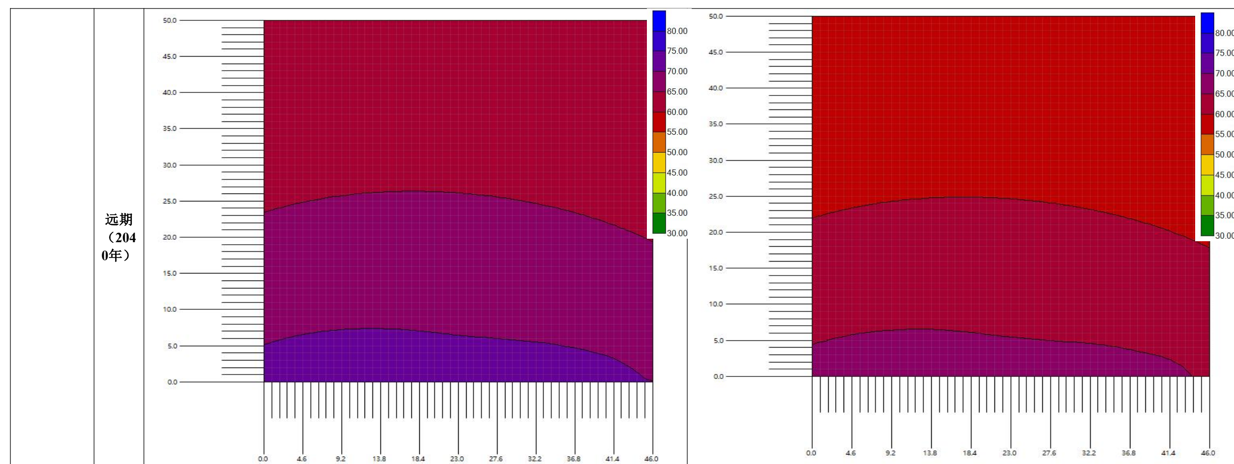
图 17 项目垂向等声级线图
