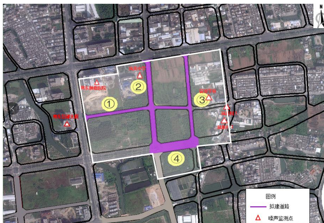
附图 5 道路 1~道路 4 声环境现状监测布点图
