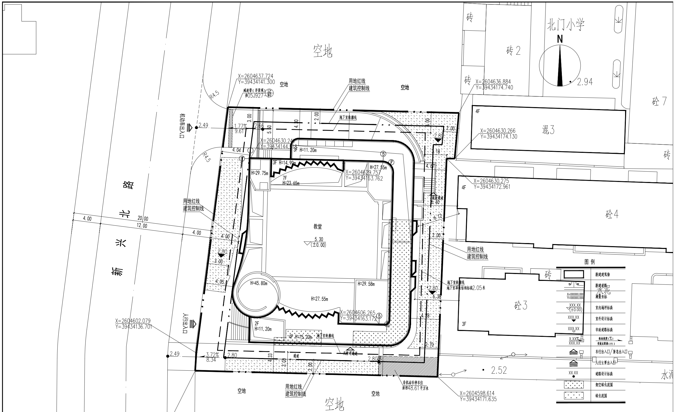
总平面图 1:200
